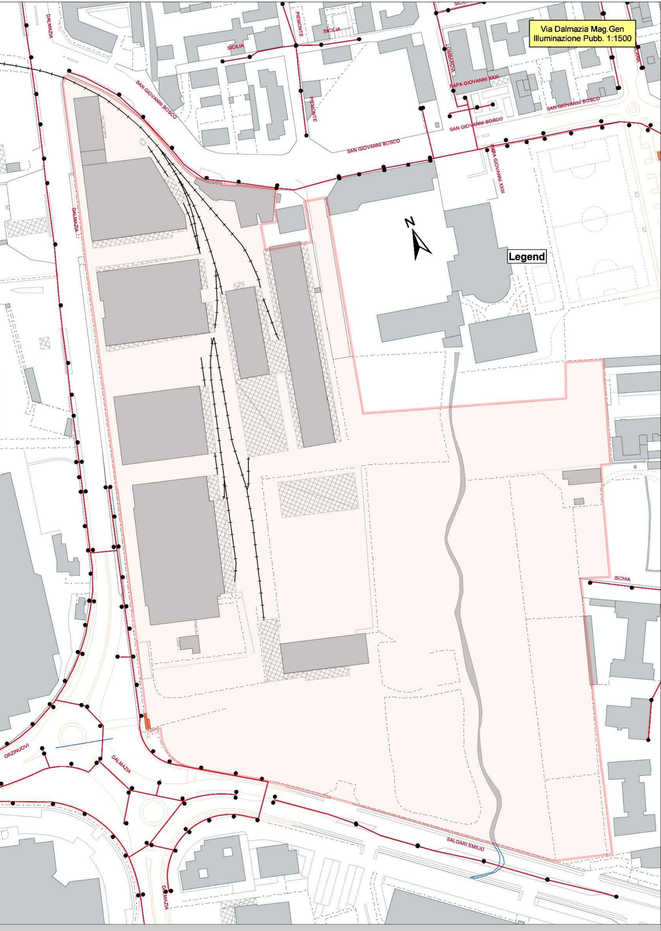
schema rete illuminazione pubblica
