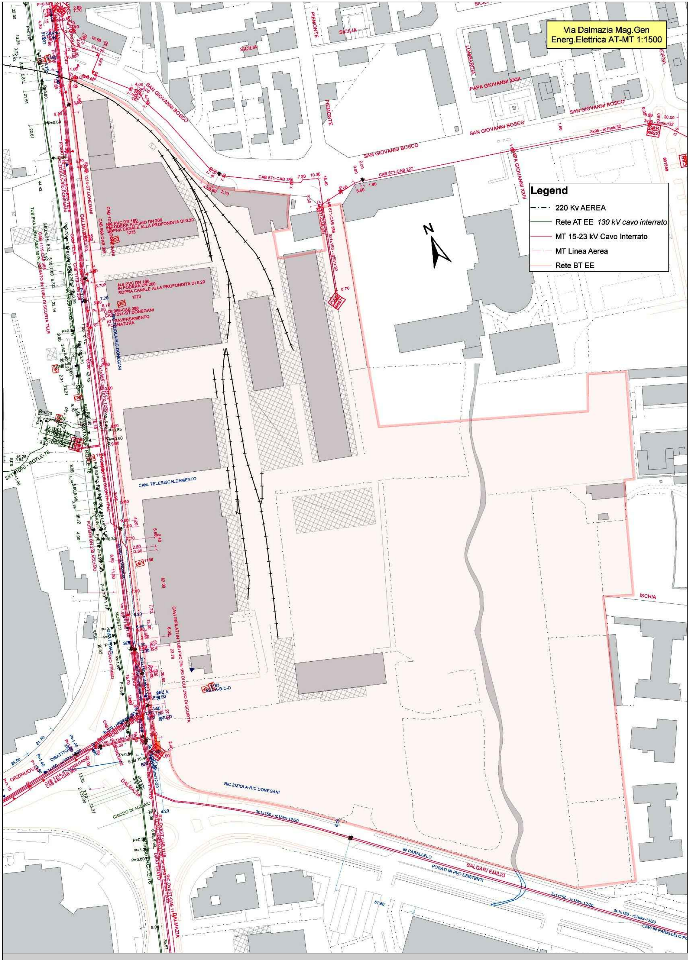
schema rete elettrica media e alta tensione
