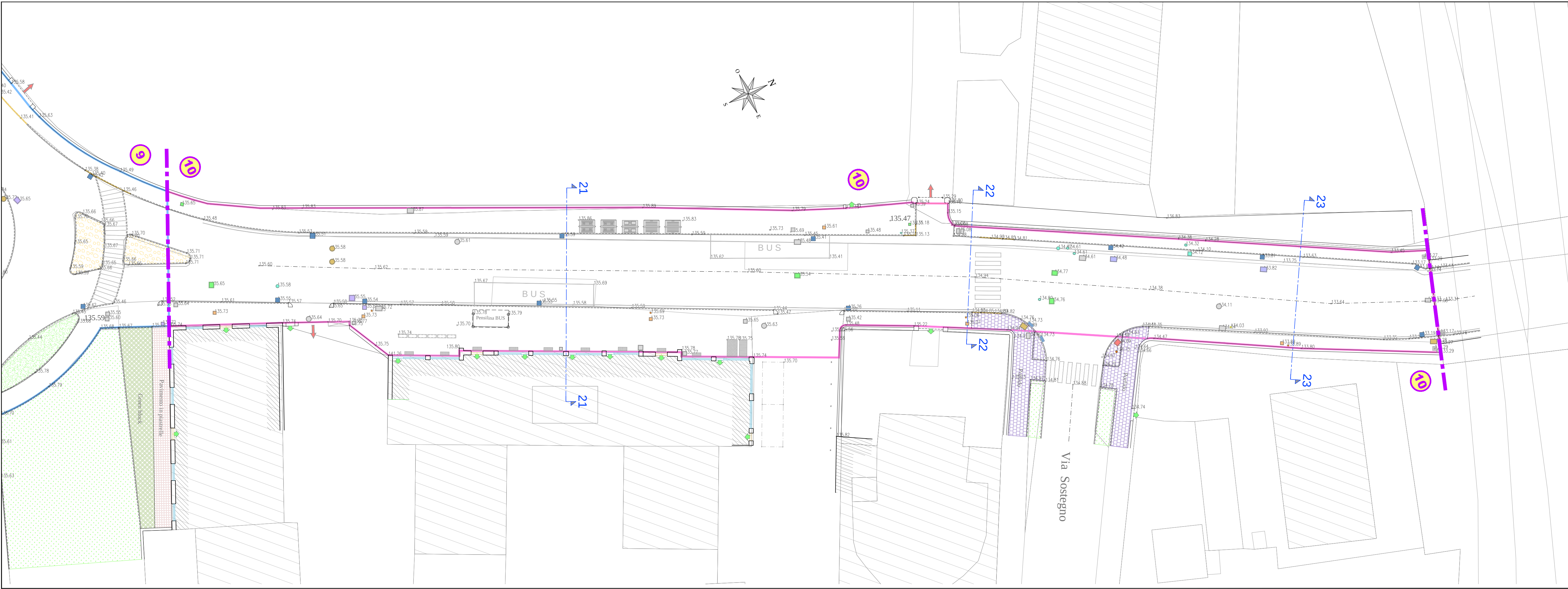
STATO DI FATTO - Via CORSICA (tratto fra intersezione via Zara/Sardegna e sottopasso ferroviario) - Intervento 10 (tavola 3 di 3)
