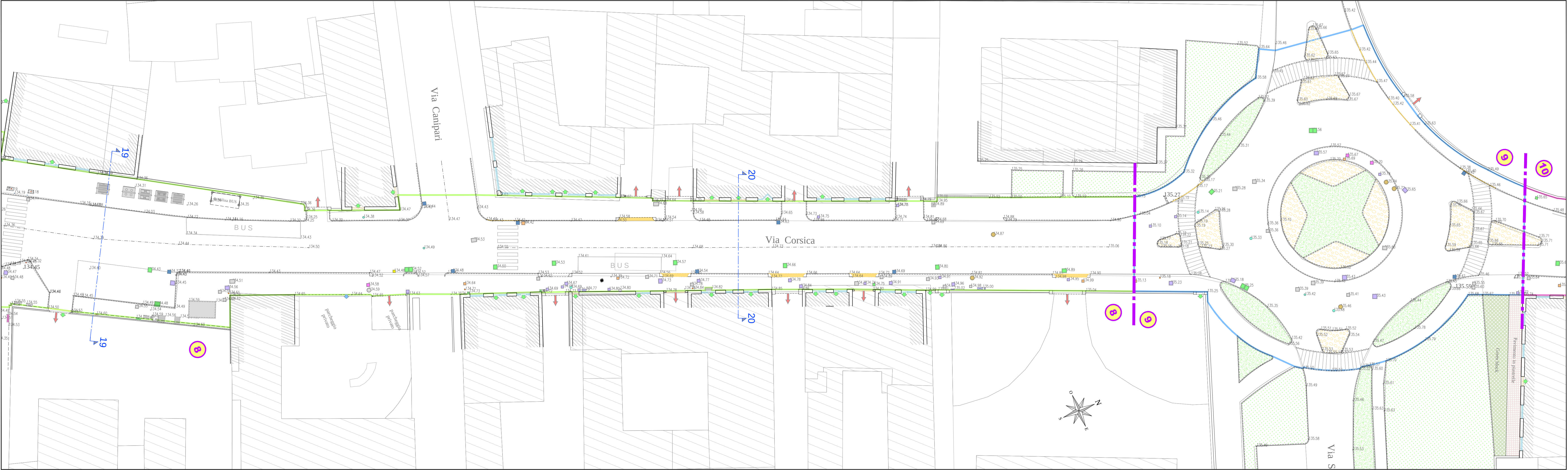
STATO DI FATTO - Via CORSICA (tratto fra intersezione via Zara/Sardegna e sottopasso ferroviario) - Intervento 10 (tavola 3 di 3)
