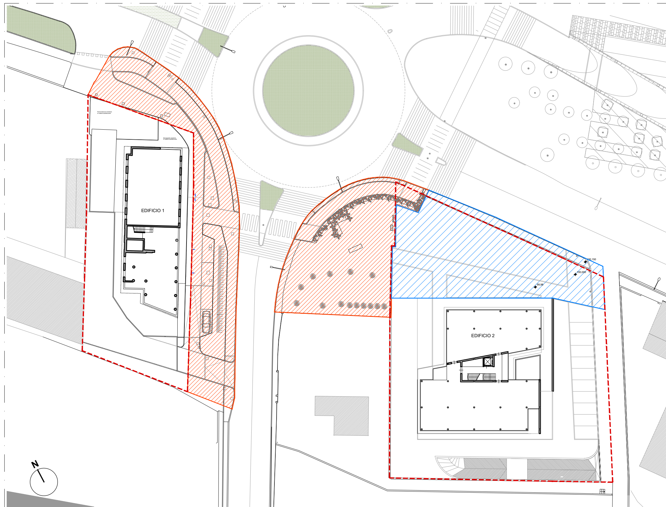
PLANIMETRIA GENERALE - REGIME DELLE OPERE - Scala 1:500
