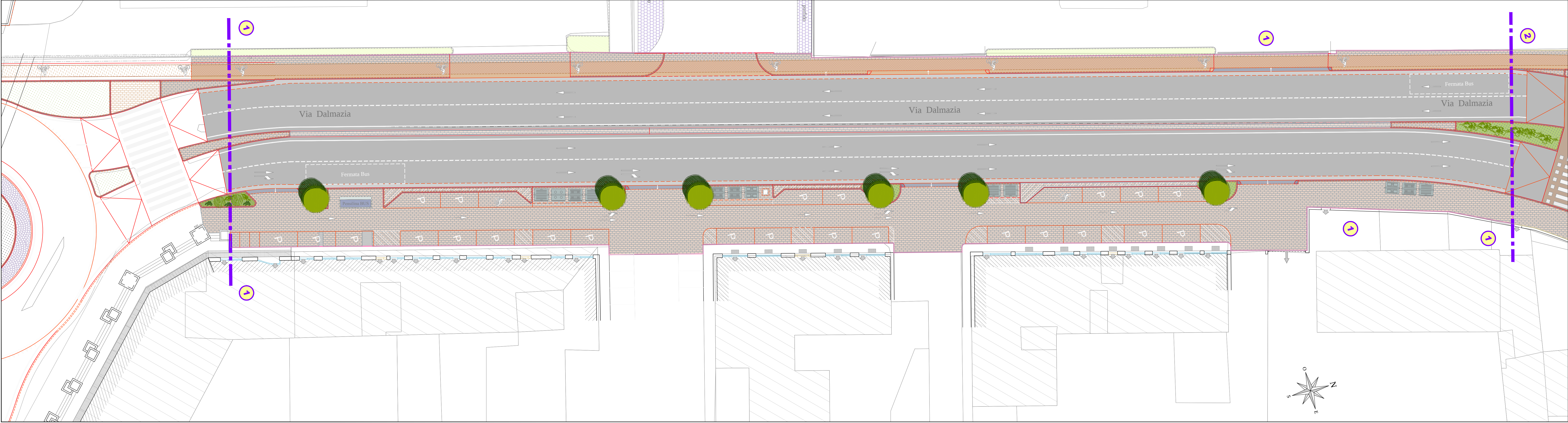
PLANIMETRIA DI PROGETTO - Via DALMAZIA ( tratto via S. Giovanni Bosco - Via Zara / Rotatoria di intersezione con Via Zara / tratto via Zara - sottopasso ferroviario) - Interventi 1/2/3 - (tavola 2 di 3)
