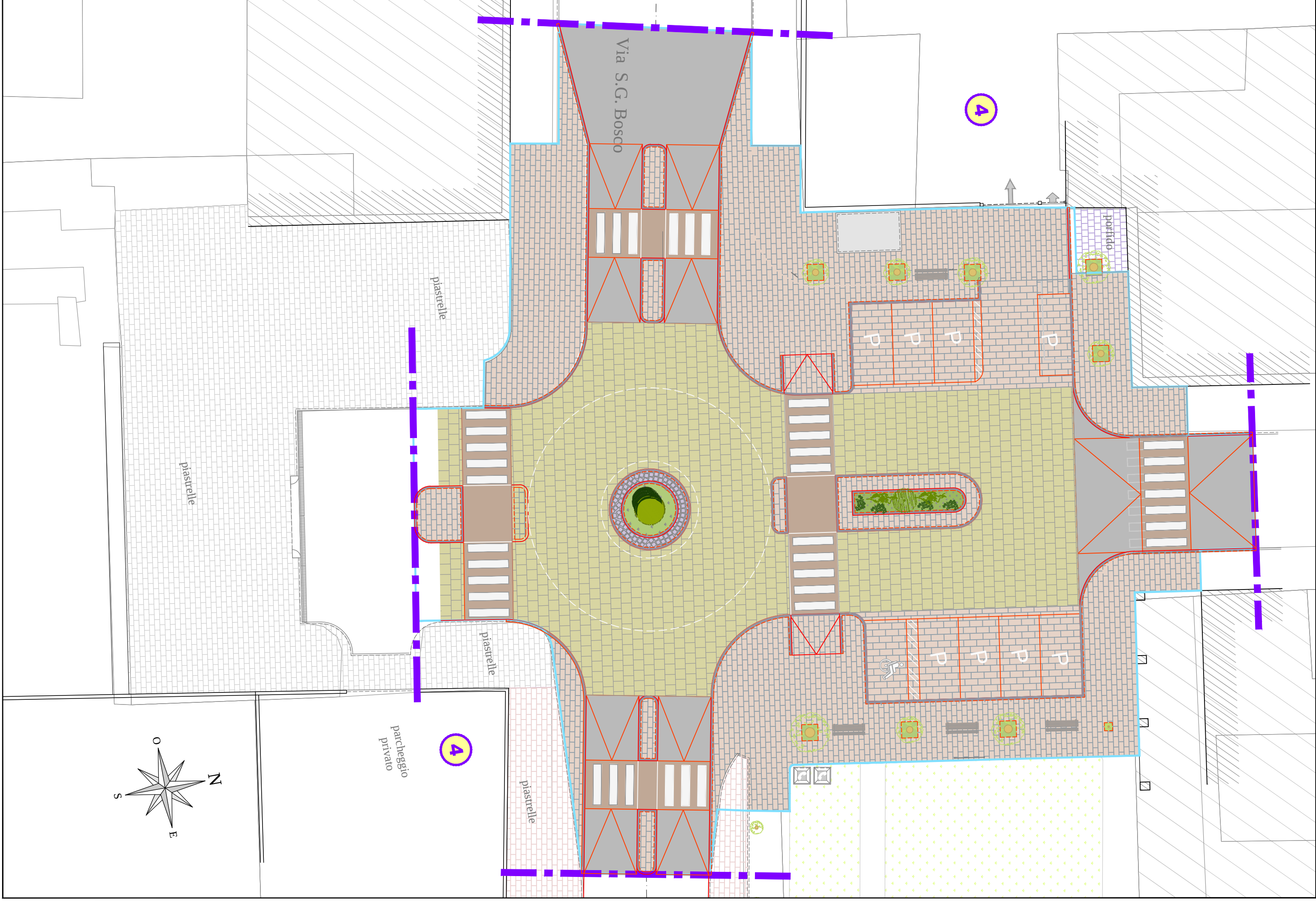
PLANIMETRIA DI PROGETTO - VIA San Giovanni BOSCO (Piazzale Papa Giovanni XXIII) - Intervento 4 (tavola 3 di 3)
