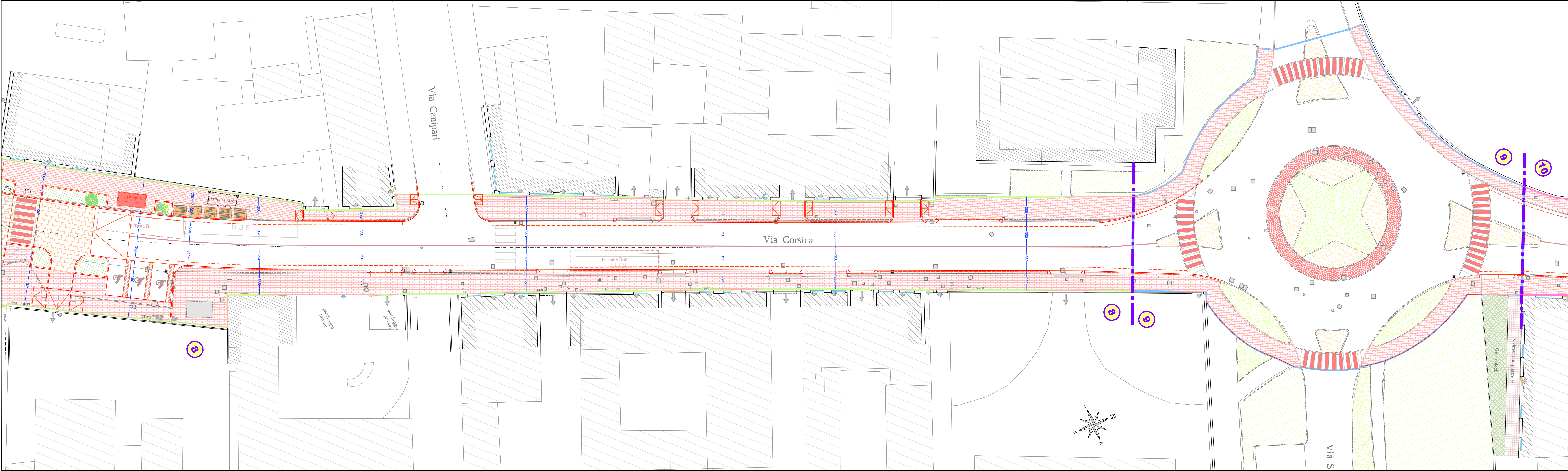
SOVRAPPOSIZIONE STATO DI FATTO E PROGETTO - Via CORSICA (tratto fra intersezione via Zara/Sardegna e sottopasso ferroviario) - Intervento 10 (tavola 3 di 3)
