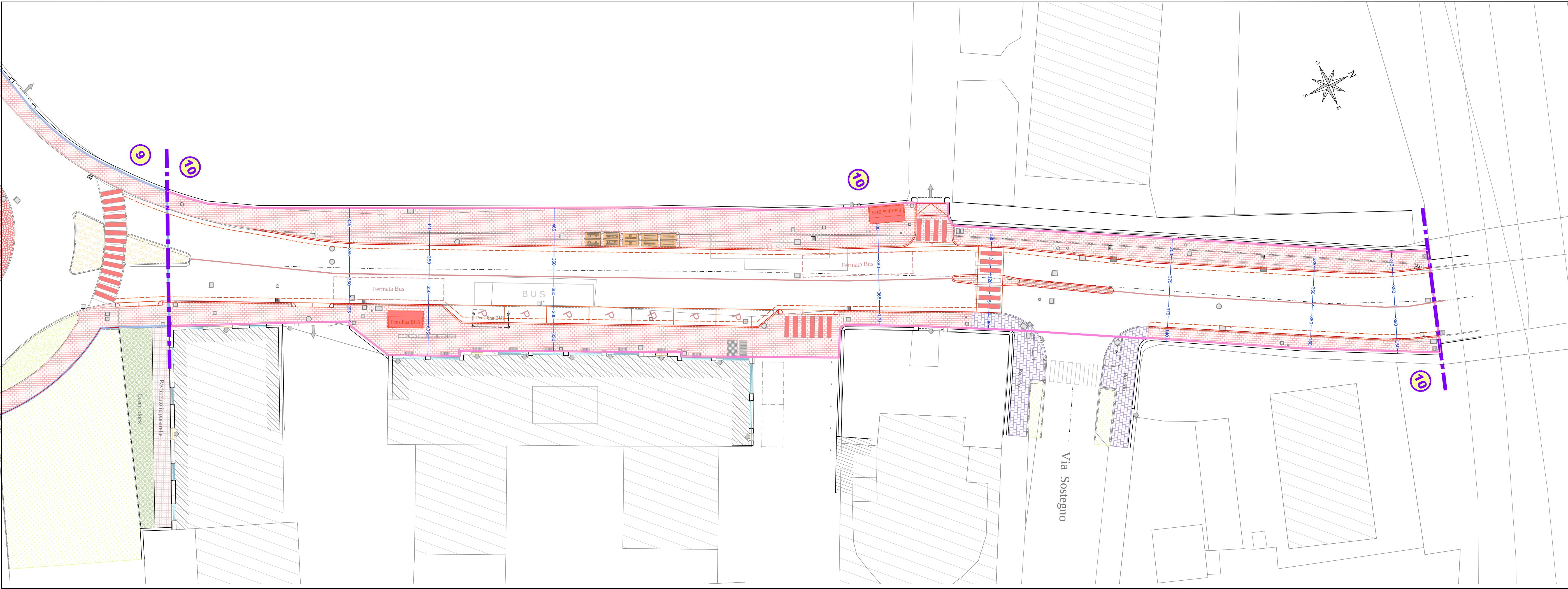
SOVRAPPOSIZIONE STATO DI FATTO E PROGETTO - Via CORSICA (tratto fra intersezione via Zara/Sardegna e sottopasso ferroviario) - Intervento 10 (tavola 3 di 3)
