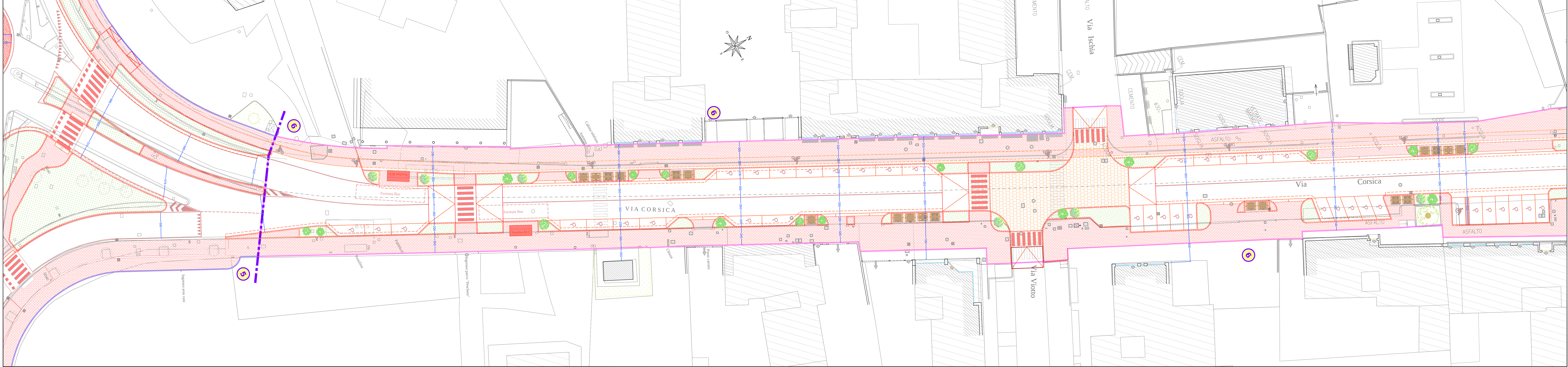
SOVRAPPOSIZIONE STATO DI FATTO E PROGETTO - Via CORSICA (tratto fra intersezione Via Salgari/Lamarmora ed intersezione via S.G. Bosco/Cefalonia) - Interventi 6/7 (tavola 3 di 3)
