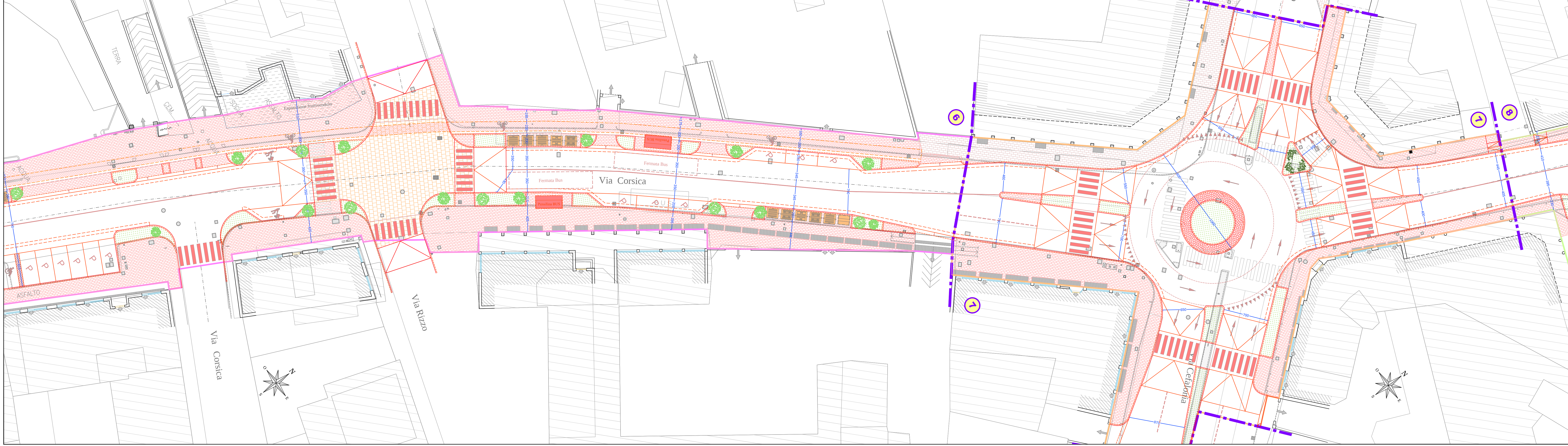
SOVRAPPOSIZIONE STATO DI FATTO E PROGETTO - Via CORSICA (tratto fra intersezione Via Salgari/Lamarmora ed intersezione via S.G. Bosco/Cefalonia) - Interventi 6/7 (tavola 3 di 3)
