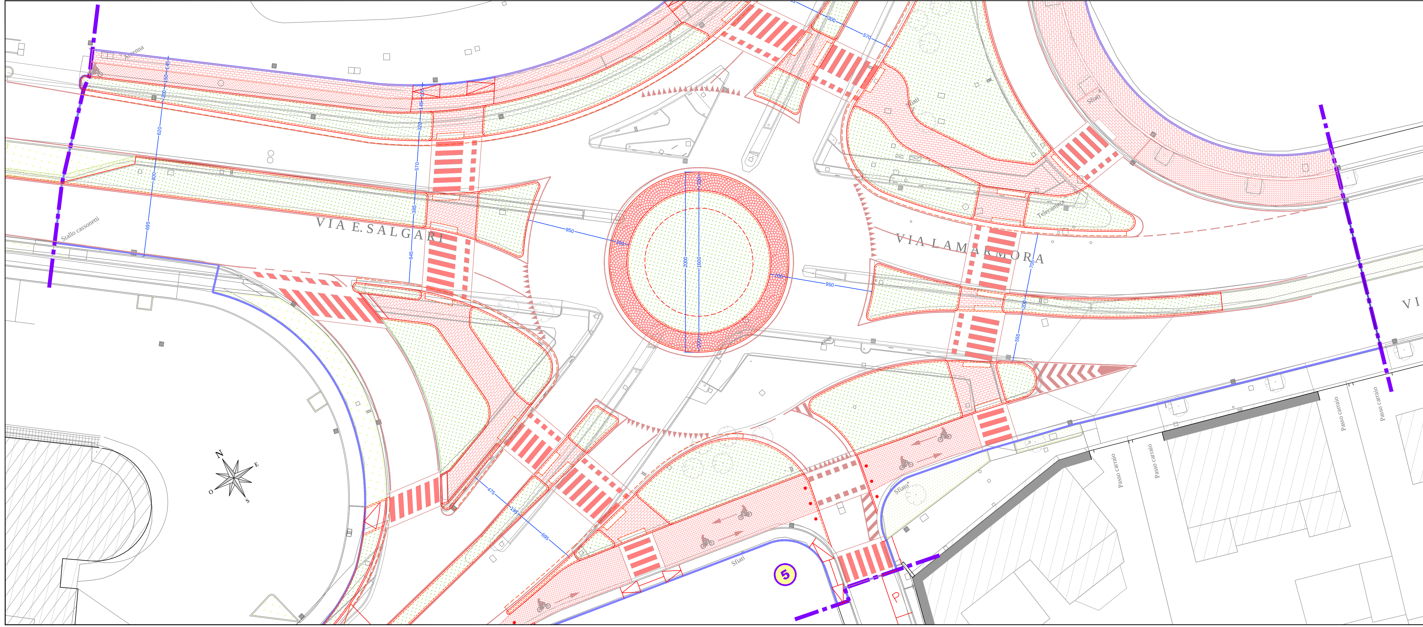
SOVRAPPOSIZIONE STATO DI FATTO E PROGETTO - Via CORSICA (tratto fra intersezione Via Salgari/Lamarmora ed intersezione via S.G. Bosco/Cefalonia) - Intervento 6 (tavola 2 di 3)
