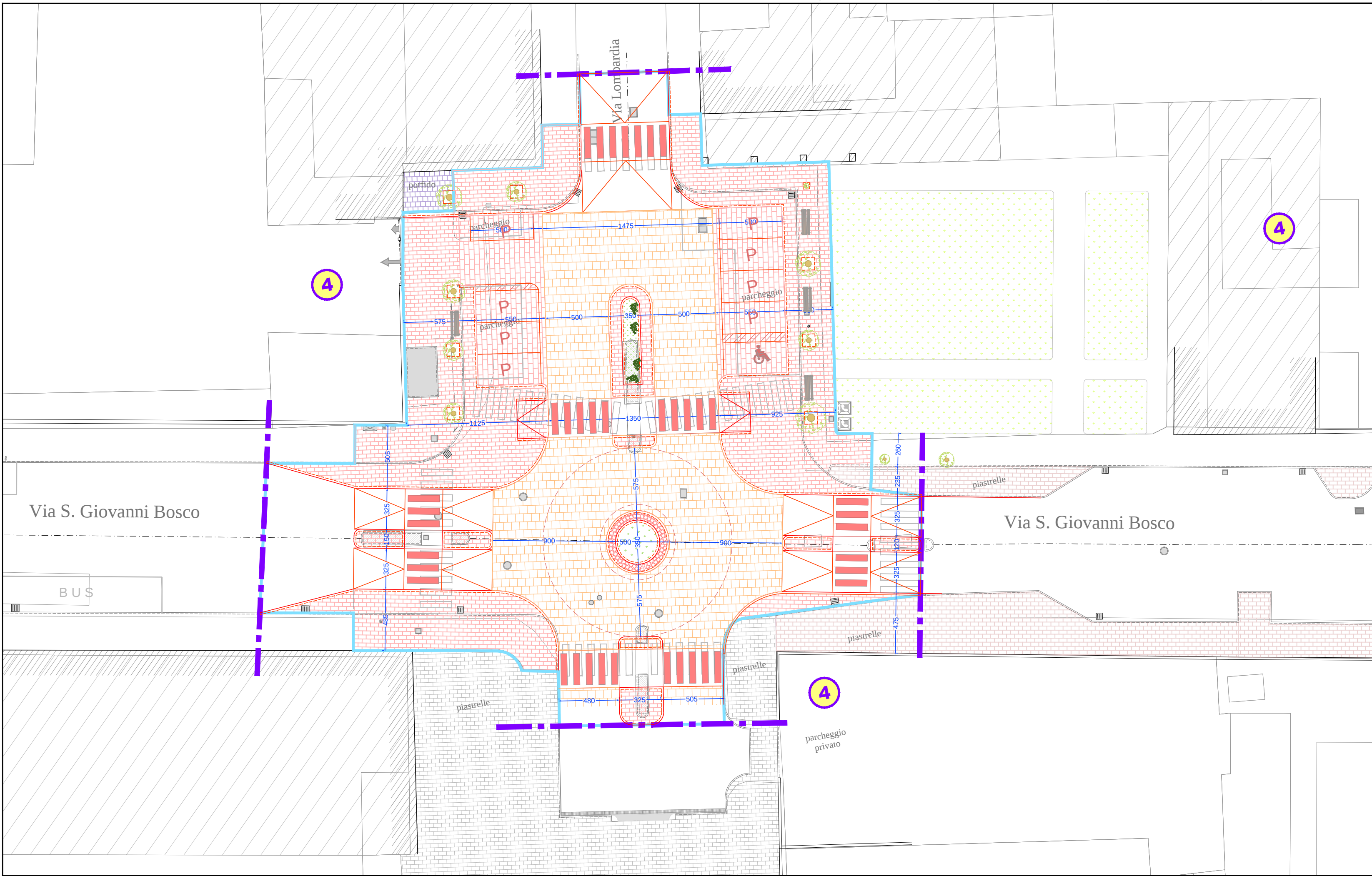
SOVRAPPOSIZIONE STATO DI FATTO E PROGETTO - VIA San Giovanni BOSCO (Piazzale Papa Giovanni XXIII) - Intervento 4 (tavola 3 di 3)
