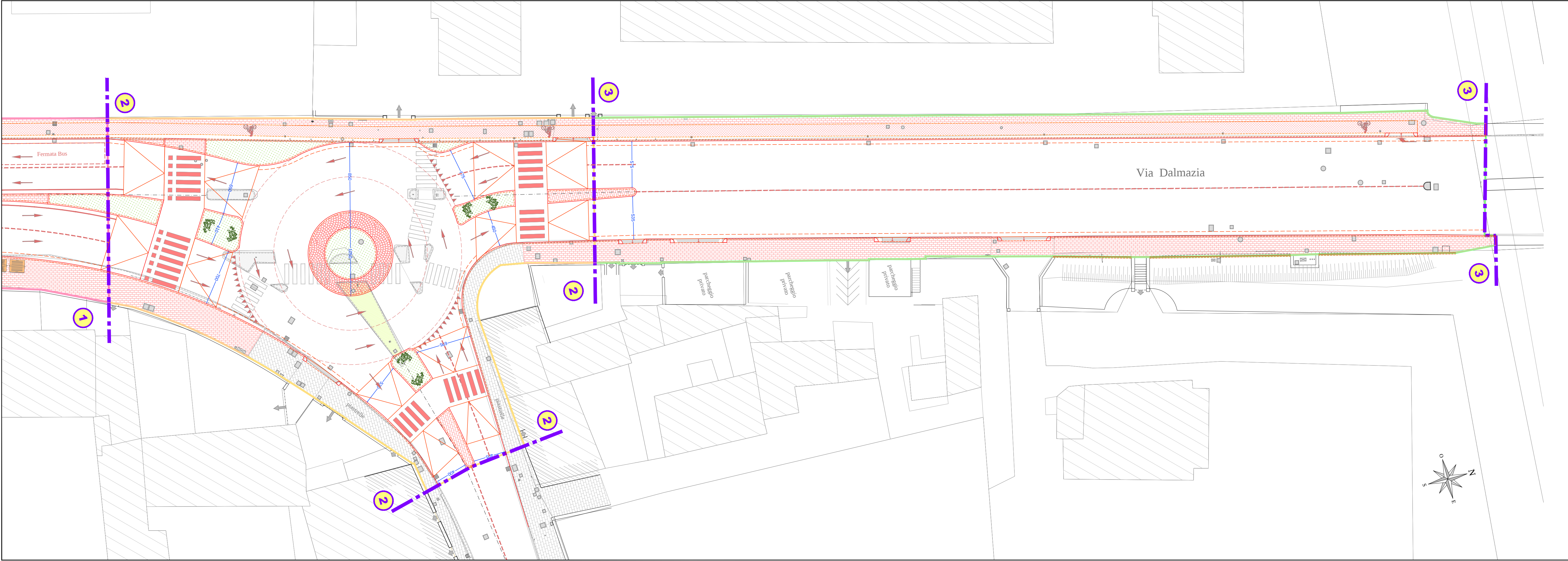
SOVRAPPOSIZIONE STATO DI FATTO E PROGETTO - VIA San Giovanni BOSCO (Piazzale Papa Giovanni XXIII) - Intervento 4 (tavola 3 di 3)
