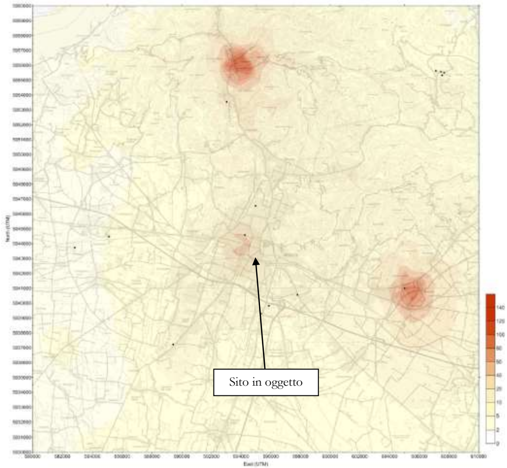
Concentrazioni medie annuali ( \mu\text{g}/\text{m}^3 ) NO x dovute alle sorgenti industriali (Concentrazione massima: 139,07 \mu\text{g}/\text{m}^3 )
