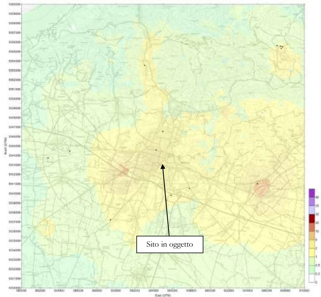
Concentrazioni medie annuali ( \mu\text{g}/\text{m}^3 ) \text{PM}_{10} dovute alle sorgenti industriali (Concentrazione massima: 7,23 \mu\text{g}/\text{m}^3 )
