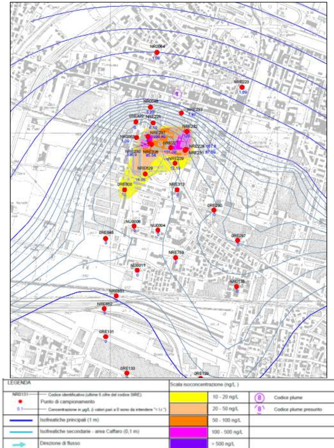
Estratto tavola 6B – Carta delle isoconcentrazioni di PCB nella prima falda – campagna di monitoraggio di ottobre 2016
