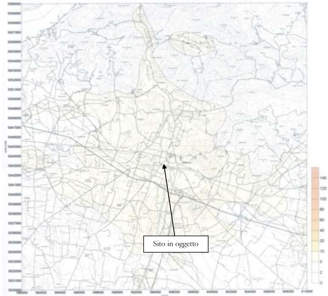
Concentrazione media annuale NOx (µg/m³) attribuita al riscaldamento civile
