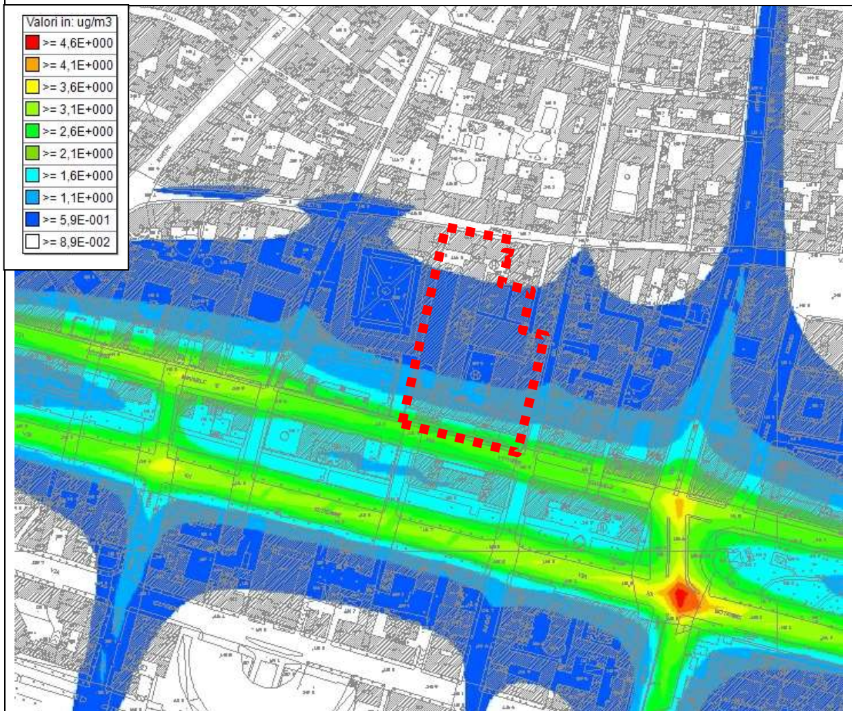
Scenario 1 - Concentrazione media annua di PM 10
