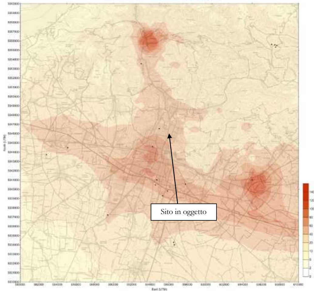
Concentrazioni medie annuali ( \mu\text{g}/\text{m}^3 ) NO x dovute a tutte le sorgenti considerate (Concentrazione massima: 165,59 \mu\text{g}/\text{m}^3 )
