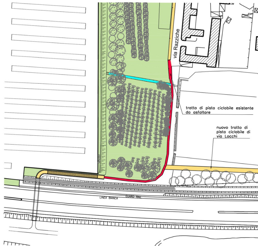
Stralcio planimetrico con tratto di pista ciclabile esistente da asfaltare.
