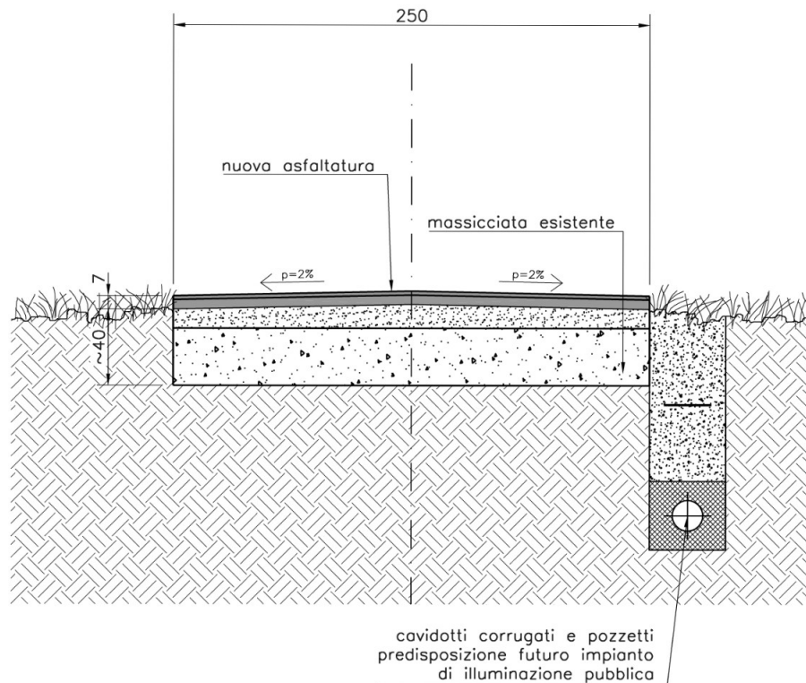
Sezione tipo tratto di pista ciclabile esistente da asfaltare.
