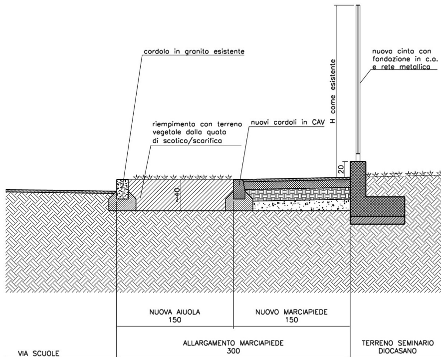
Sezione tipo di progetto.
