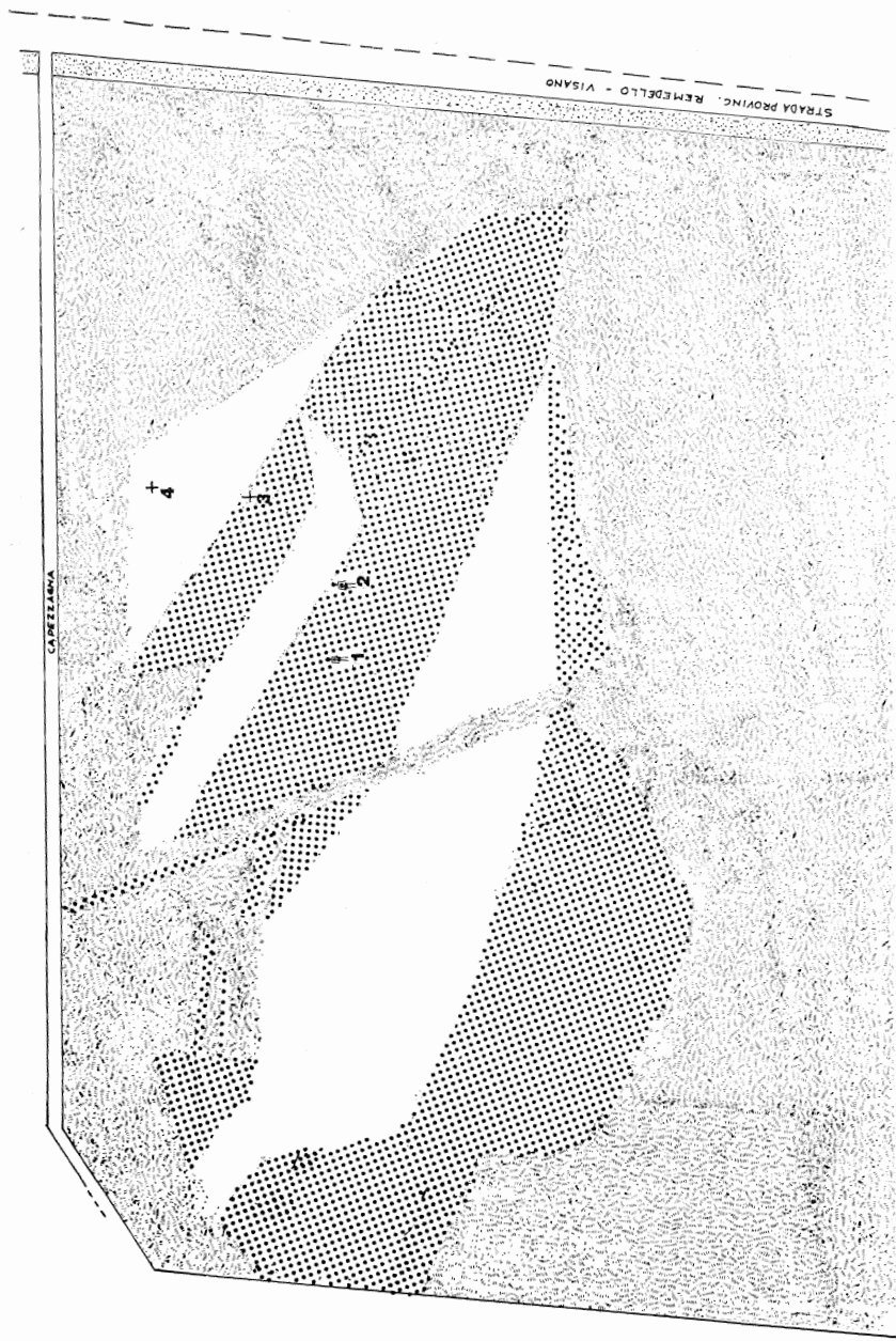
C. Tagliate-Remedello Sopra - scavi off. 1976 - all.n.5 Rilievo stratigrafico omiz. alla superficie RILEVI: AKH, MAZZOTTI LUCIANO & GEOM. SAVANI ALESSANDRO - DISEGNI: MAZZOTTI L., PERINI RINO. □ Sabbia - sc.:1: 250 ▨ Ghiala ▩ Terr. argilloso
