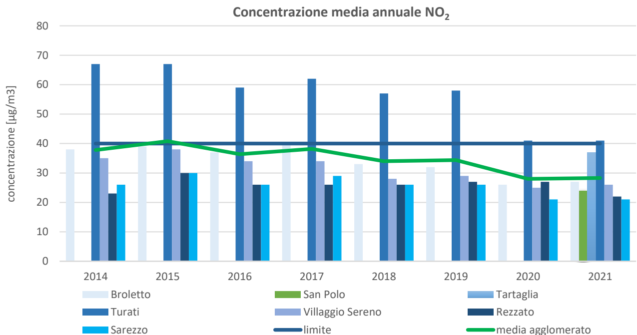
Figura 14: Concentrazioni medie annuali di NO 2 dal 2014 al 2021
