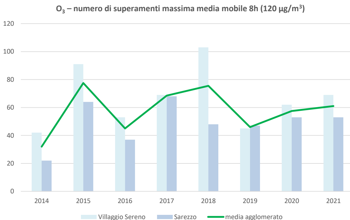
Figura 16 – Giorni di superamento del valore obiettivo per l'ozono dal 2014 al 2021.
