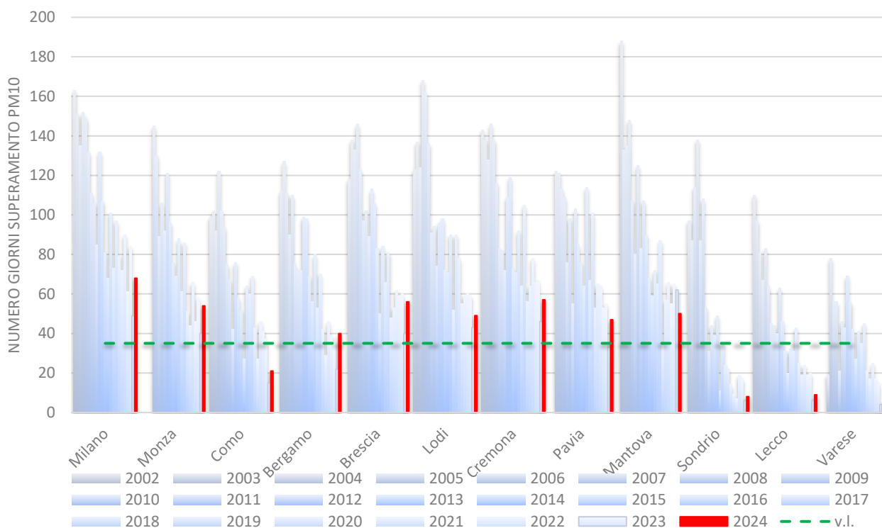
Figura 12: PM10 – Numero di giorni di superamento della soglia di 50 \mu\text{g}/\text{m}^3 in ciascun anno nella stazione peggiore del programma di valutazione di ogni capoluogo
