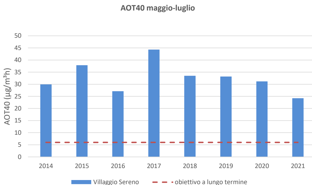
Figura 17 – AOT40 per il periodo maggio – luglio.
