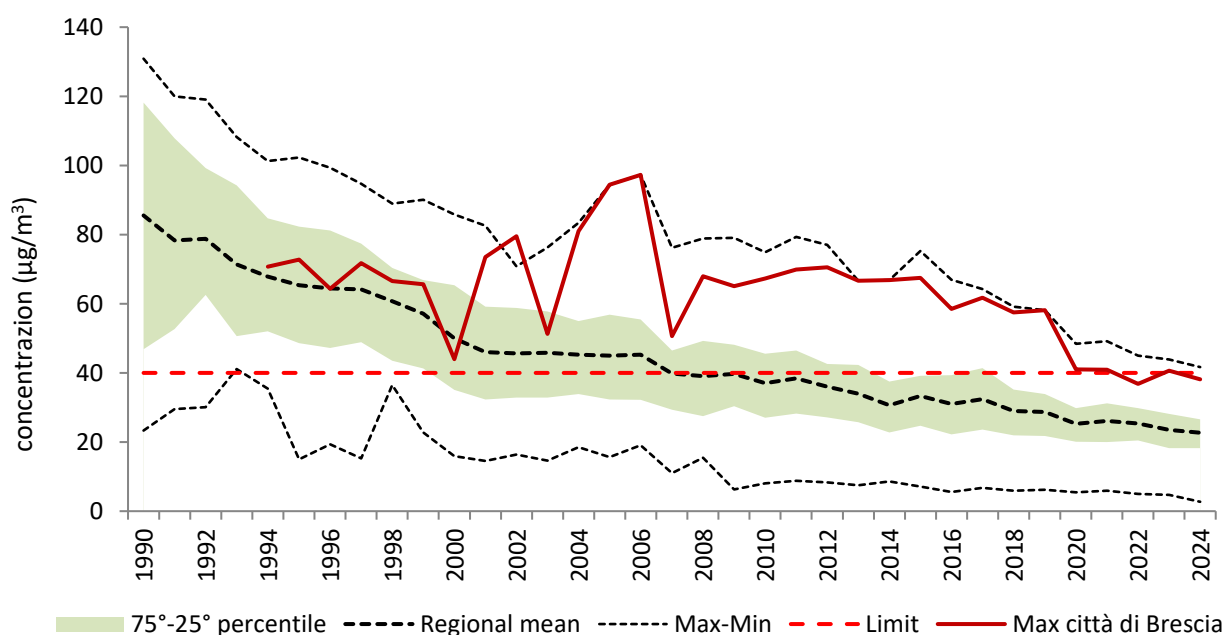
Figura 13 – Andamento delle concentrazioni medie annuali di NO 2 della Regione confrontato con il trend della città di Brescia (concentrazione annuale massima) (fonte ARPA Lombardia)
