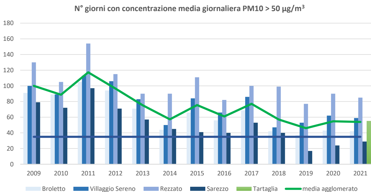
Figura 9: Numero di giorni caratterizzati da una concentrazione media giornaliera di PM10 > 50 µg/m³
