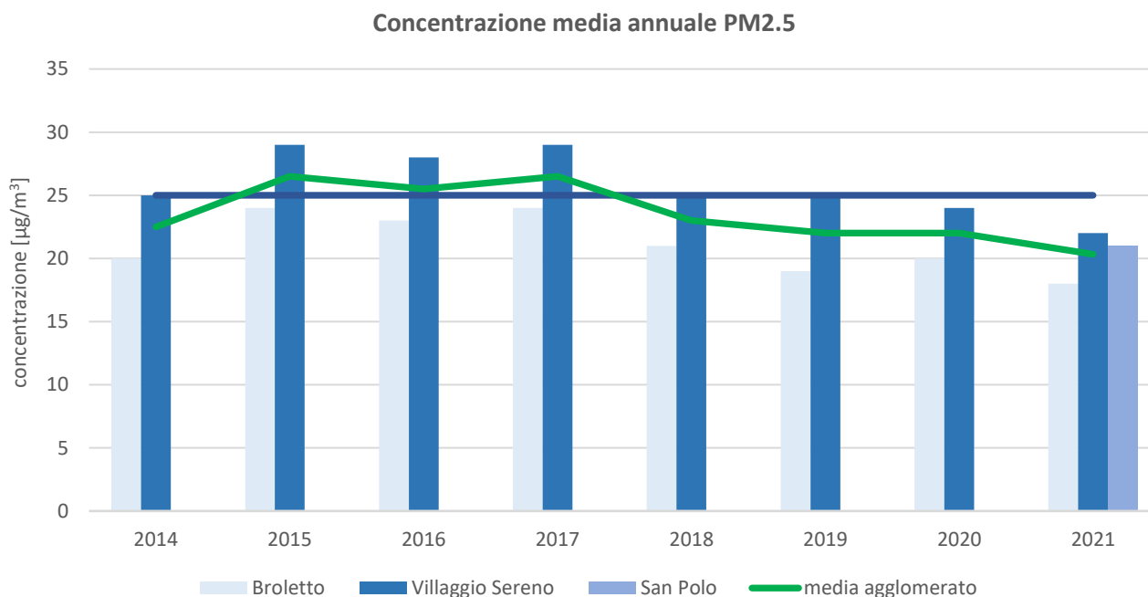
Figura 10: Concentrazioni medie annuali di PM2.5 dal 2014 al 2021
