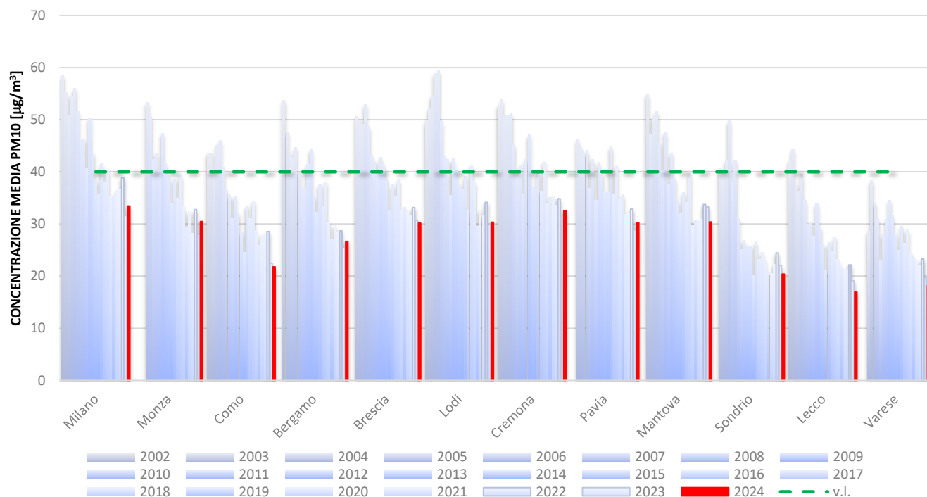
Figura 11: PM10 – Medie annue in \mu\text{g}/\text{m}^3 nella stazione peggiore del programma di valutazione di ogni capoluogo. (fonte ARPA Lombardia)
