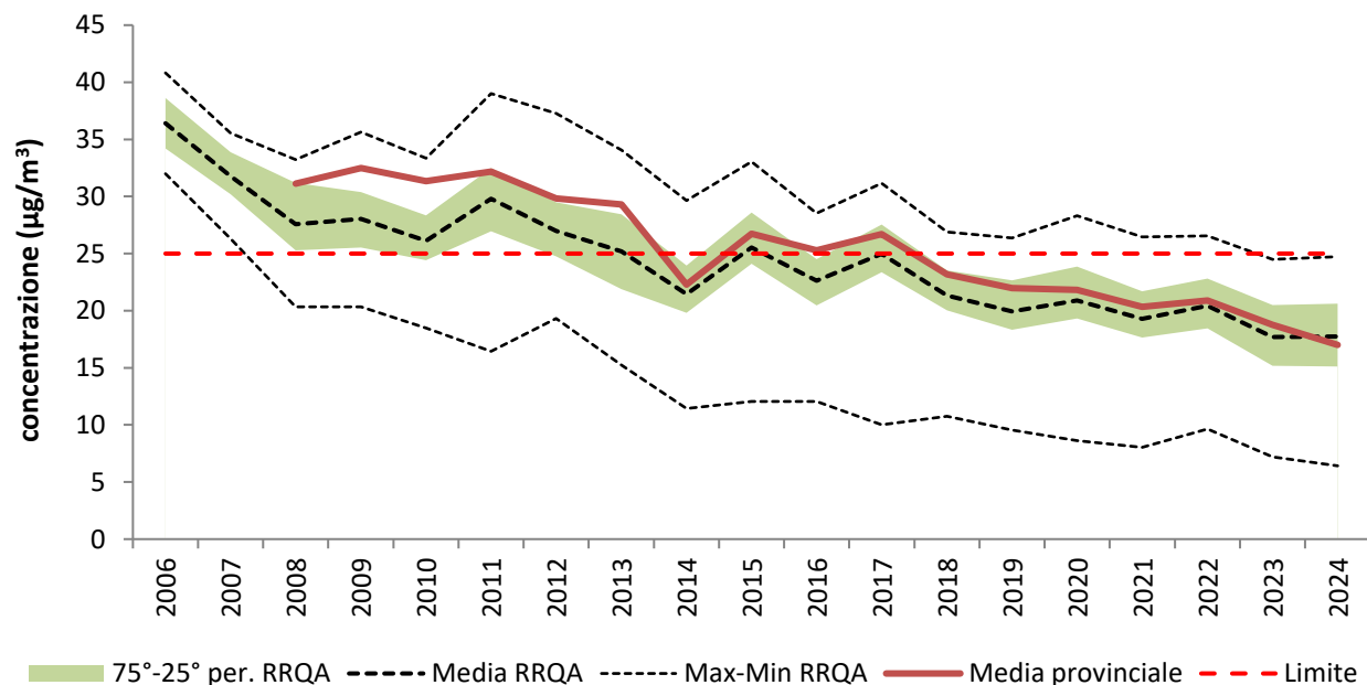
Figura 7: Andamento delle concentrazioni medie annuali di PM2.5 della Regione confrontato con il trend della Provincia di Brescia (fonte ARPA Lombardia)
