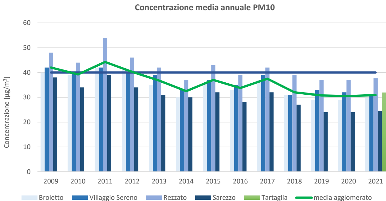
Figura 8: Grafico dei valori concentrazioni medie annuali di PM10 dal 2009 al 2021
