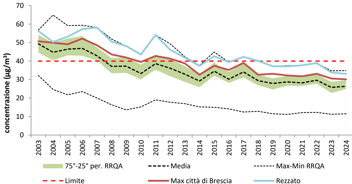
Figura 6: Andamento delle concentrazioni medie annuali di PM10 della Regione confrontato con il trend della Città di Brescia (massimo tra le stazioni) e Rezzato (fonte ARPA Lombardia)
