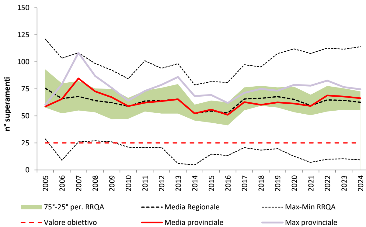
Figura 15: Andamento del numero di superamenti di O 3 (media su tre anni) della Regione confrontato con il trend della provincia di Brescia e con il massimo della provincia (fonte ARPA Lombardia).
