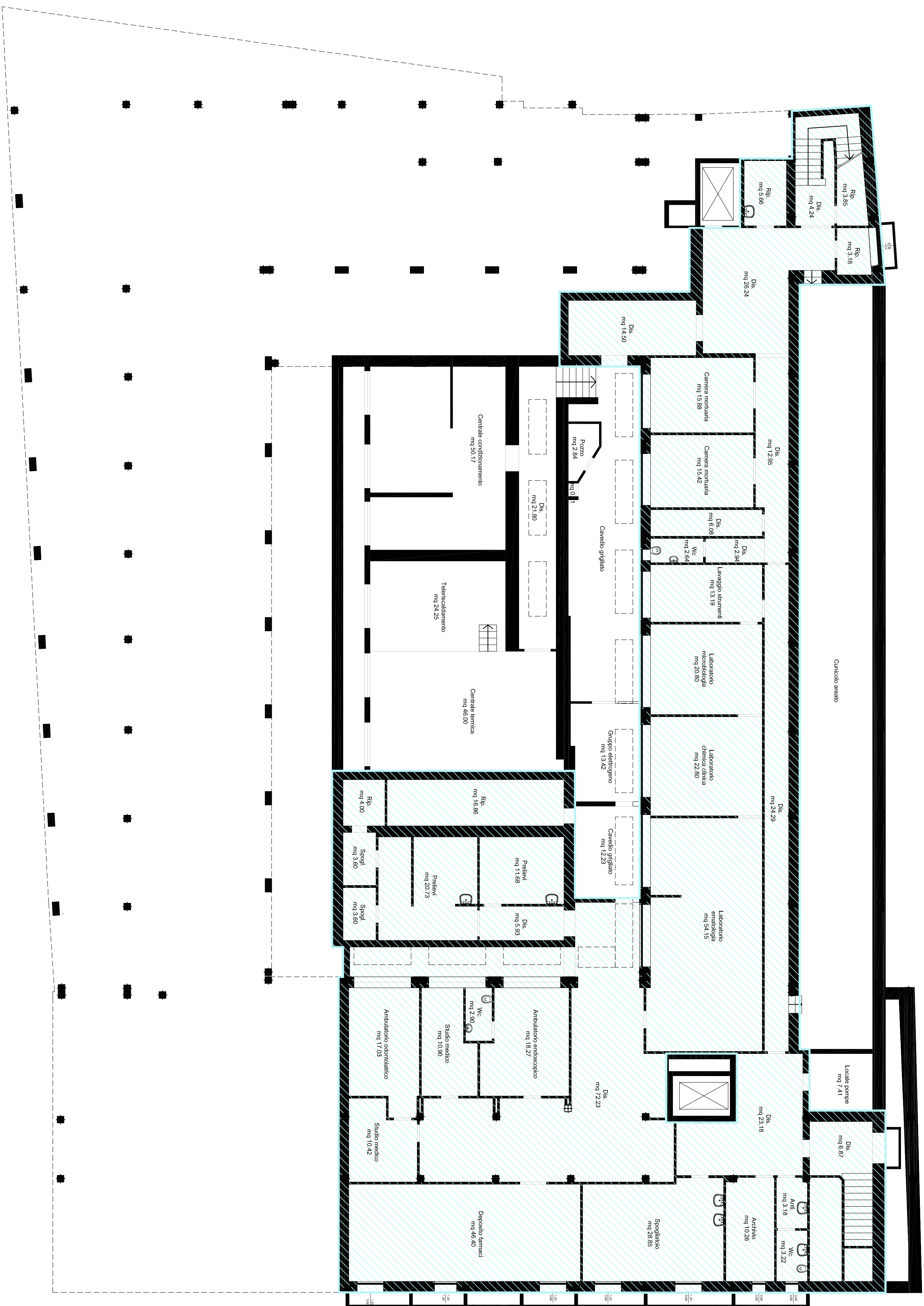
PIANTA PIANO INTERRATO 2
