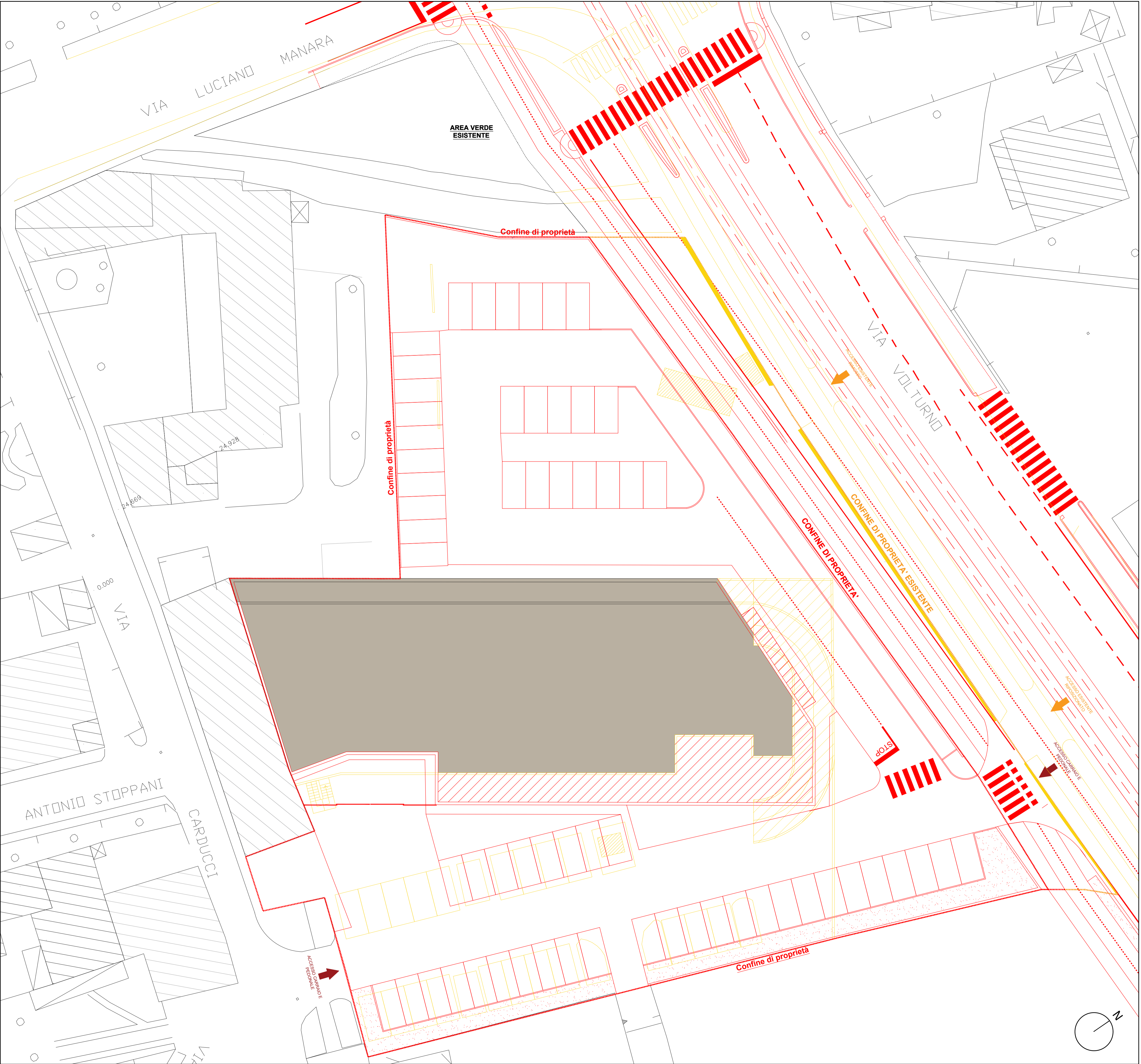
PLANIMETRIA GENERALE DI RAFFRONTO - scala 1:200
