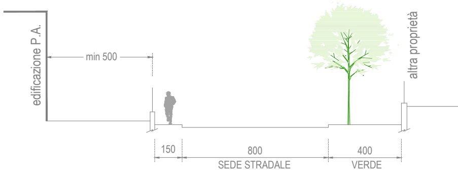
SEZIONE SCHEMATICA 1-1
