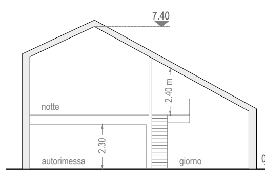
Tipologia A sezione tipo
