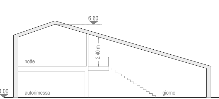
Tipologia B sezione tipo
