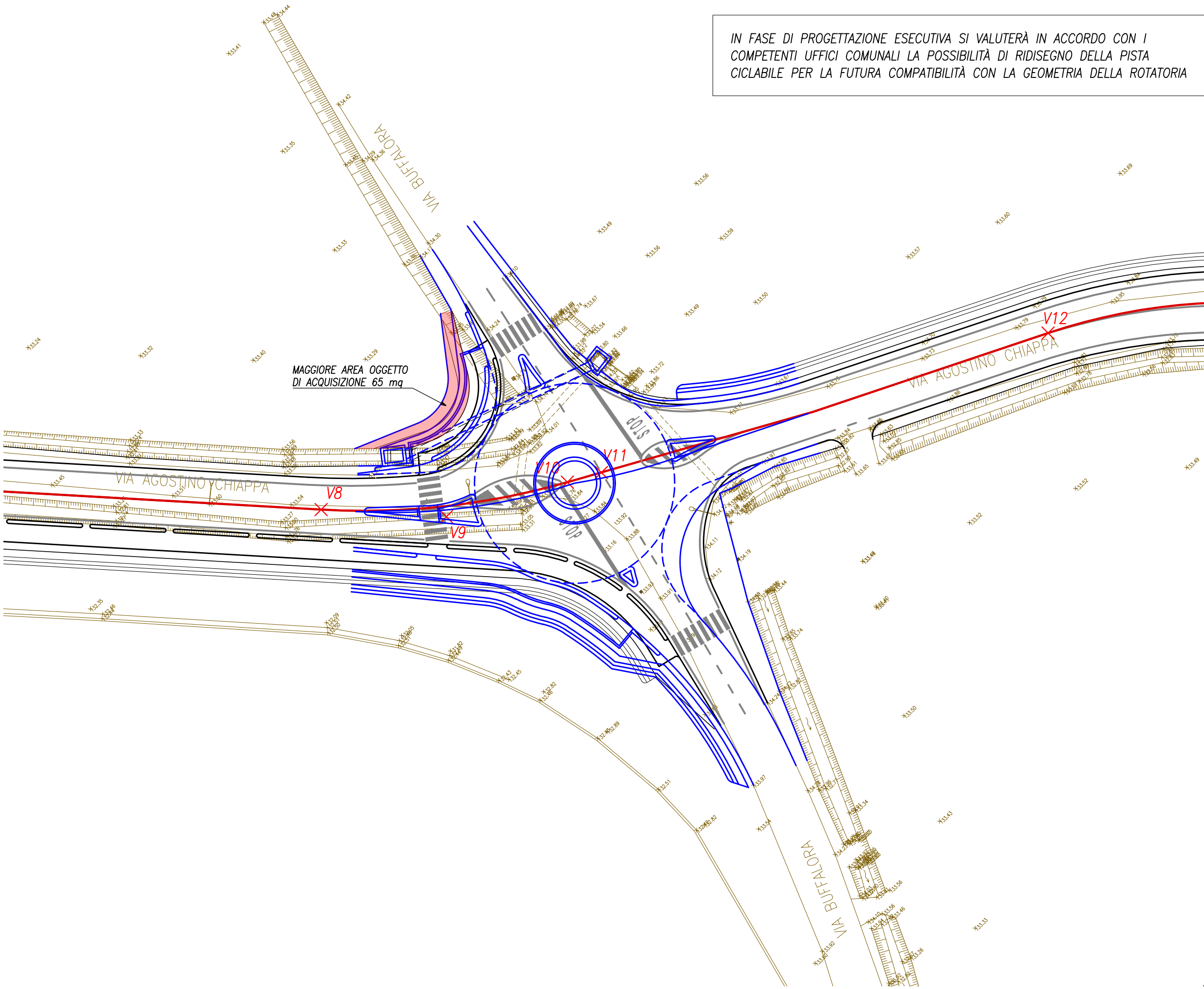
INTERSEZIONE VIA CHIAPPA/VIA BUFFALORA: SOLUZIONE CON ROTATORIA
