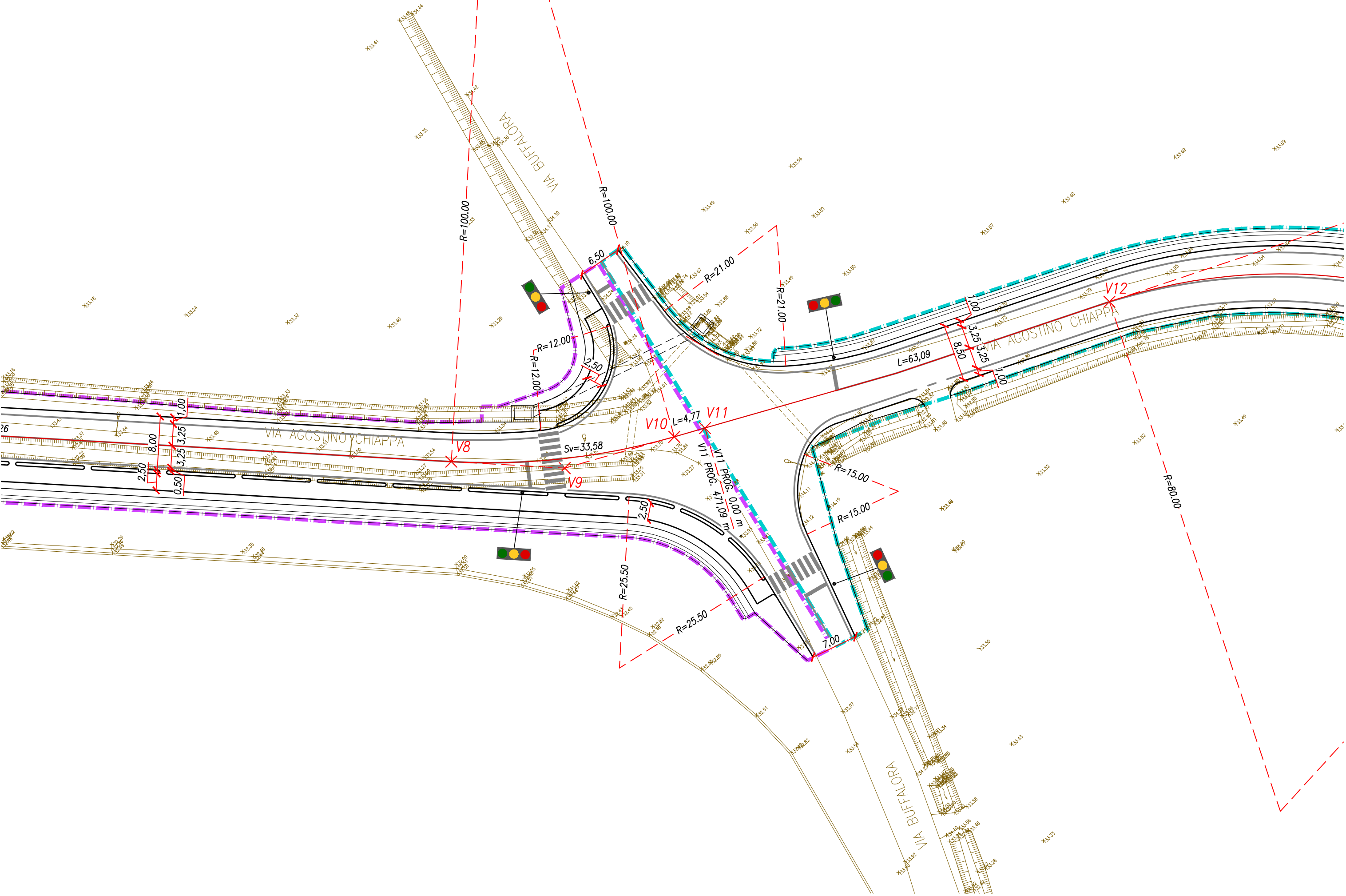
INTERSEZIONE VIA CHIAPPA/VIA BUFFALORA: SOLUZIONE CON IMPIANTO SEMAFORICO
