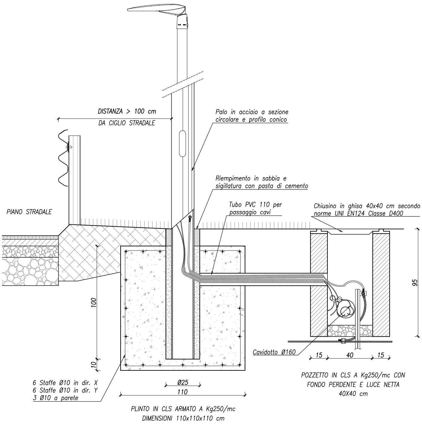
SEZIONE TIPO CAVIDOTTO LINEA IP
