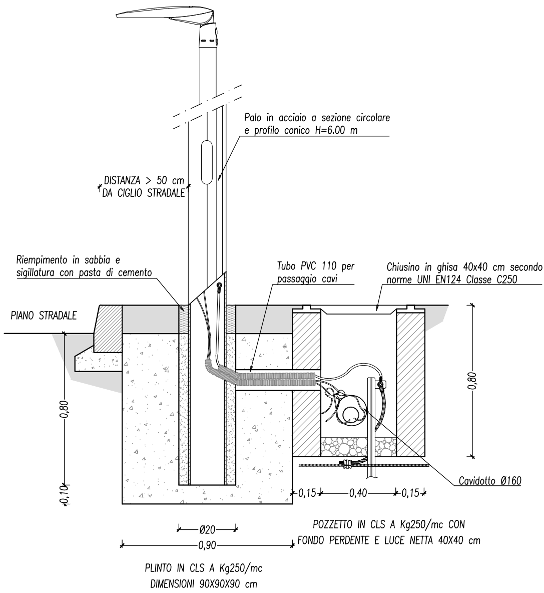
PARTICOLARE PLINTO E POZZETTO IP – ATTRAVERSAMENTO PEDONALE 1:20
