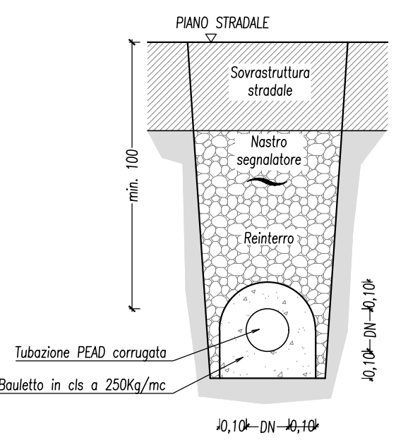
SEZIONE TIPO CAVIDOTTO LINEA IP 1:20
