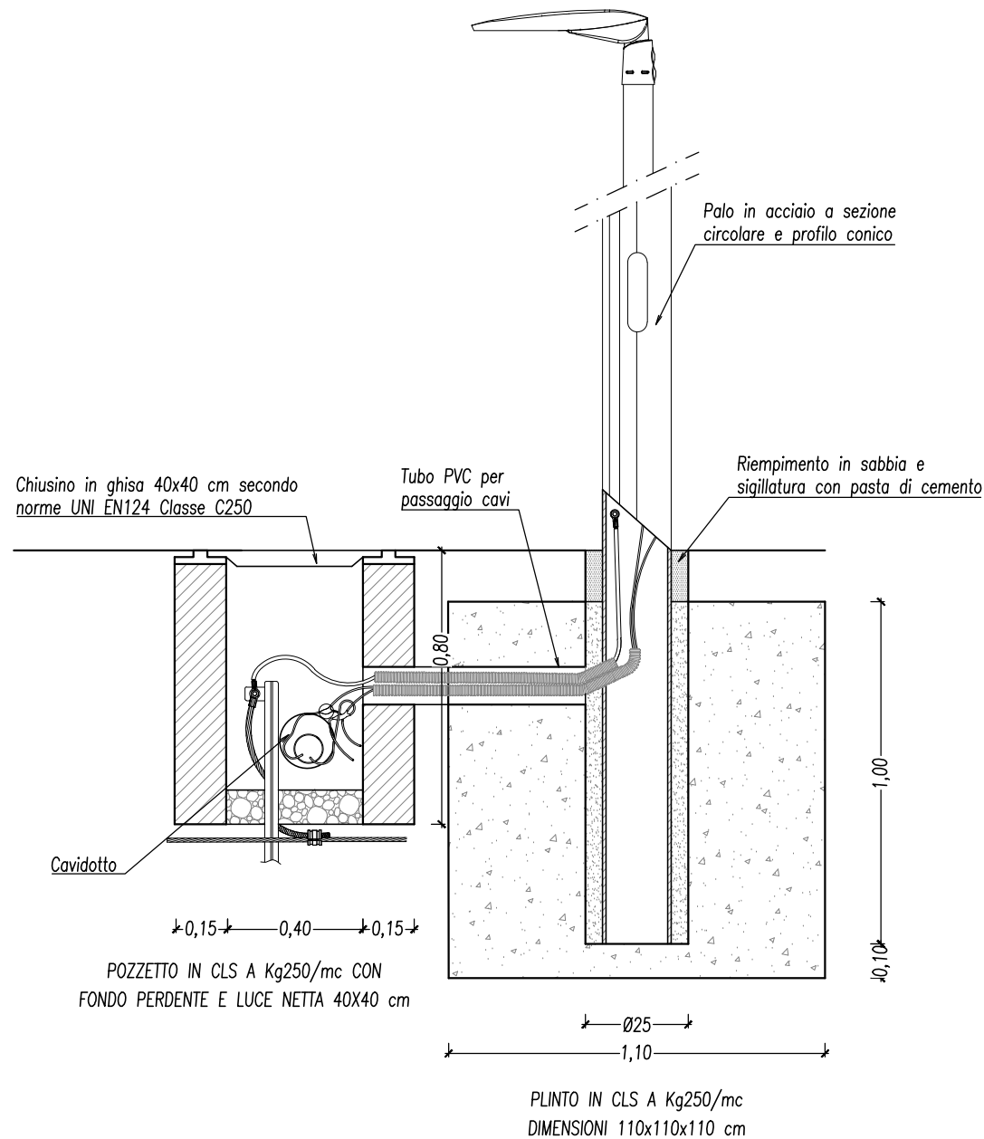
PARTICOLARE PLINTO E POZZETTO IP – ILLUMINAZIONE STRADALE 1:20
