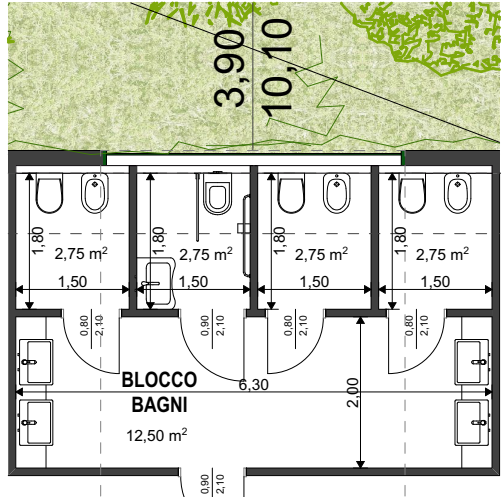
DETTAGLIO BLOCCO BAGNI 1:100
