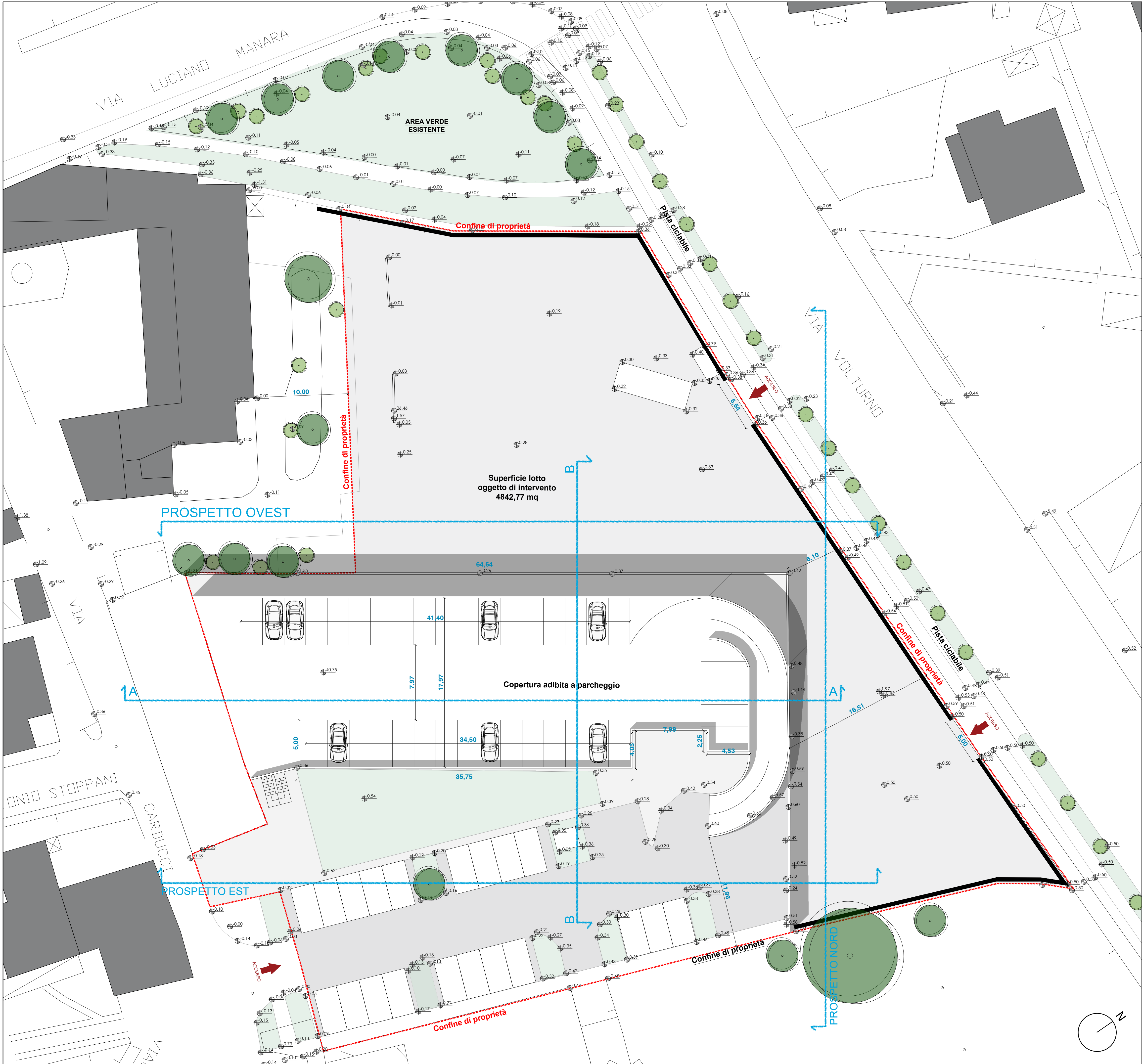
PLANIMETRIA GENERALE DI RILIEVO - scala 1:200
