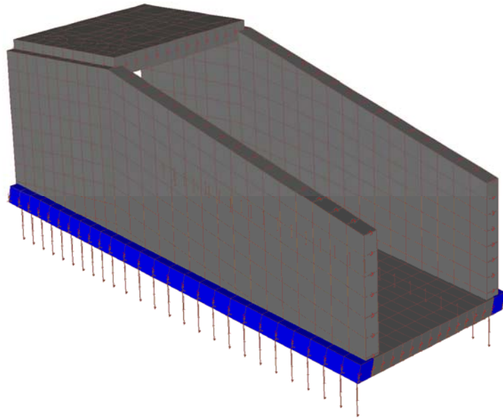
Condizione di carico n°10 (in colore blu le superfici della platea caricate)
