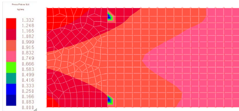
Involuppo Combinazioni agli SLU – pressioni sulla platea di fondazione (statiche)
