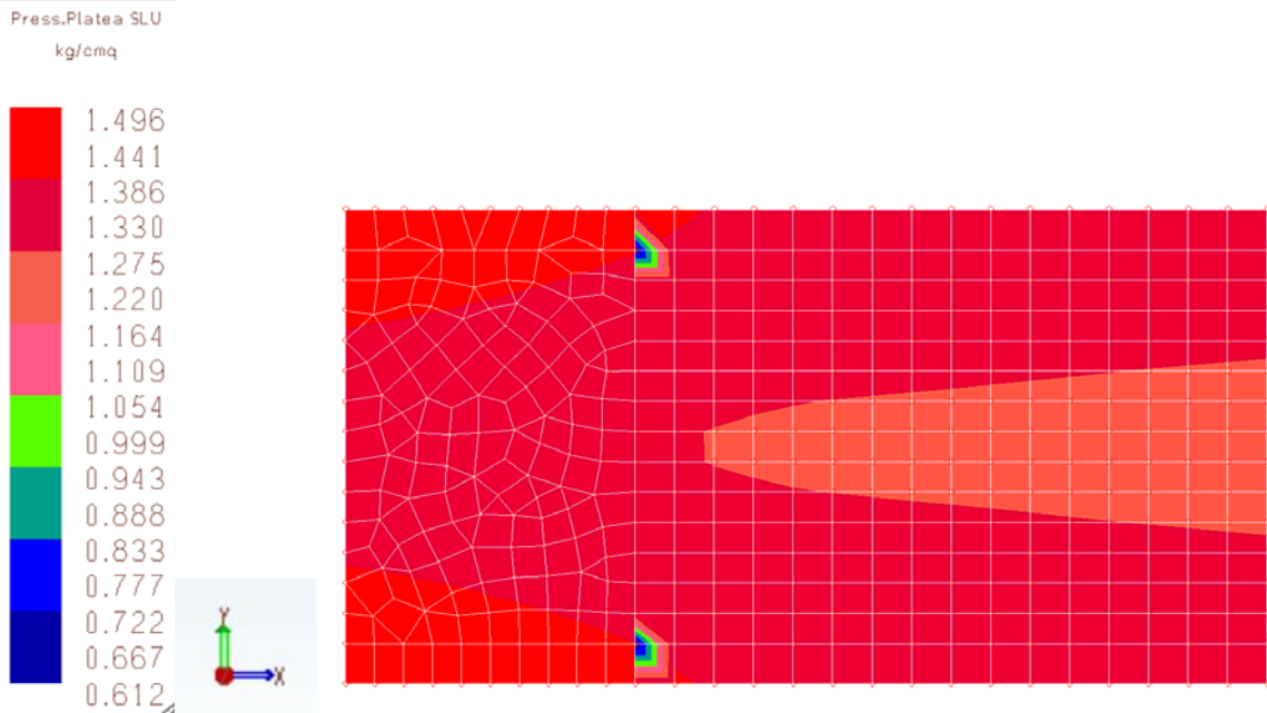
Involuppo Combinazioni agli SLV – pressioni sulla platea di fondazione (sismiche)
