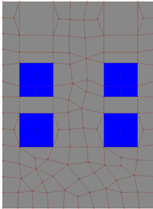
Condizione di carico n°4 (in colore blu le superfici della soletta caricate)
