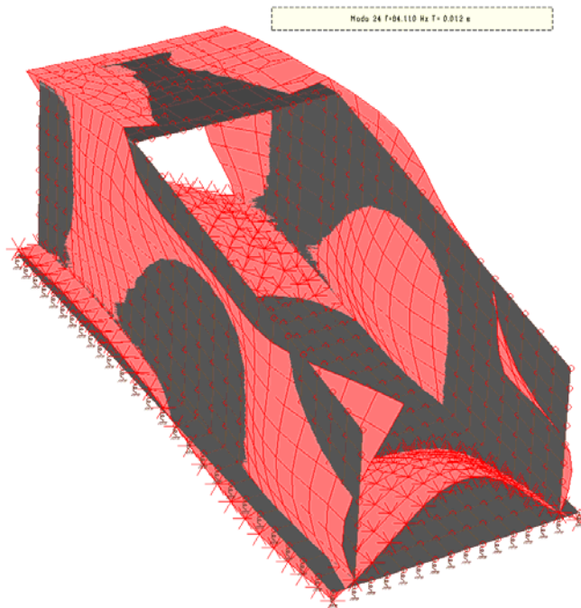
24° Modo di vibrare – principale in x-x
