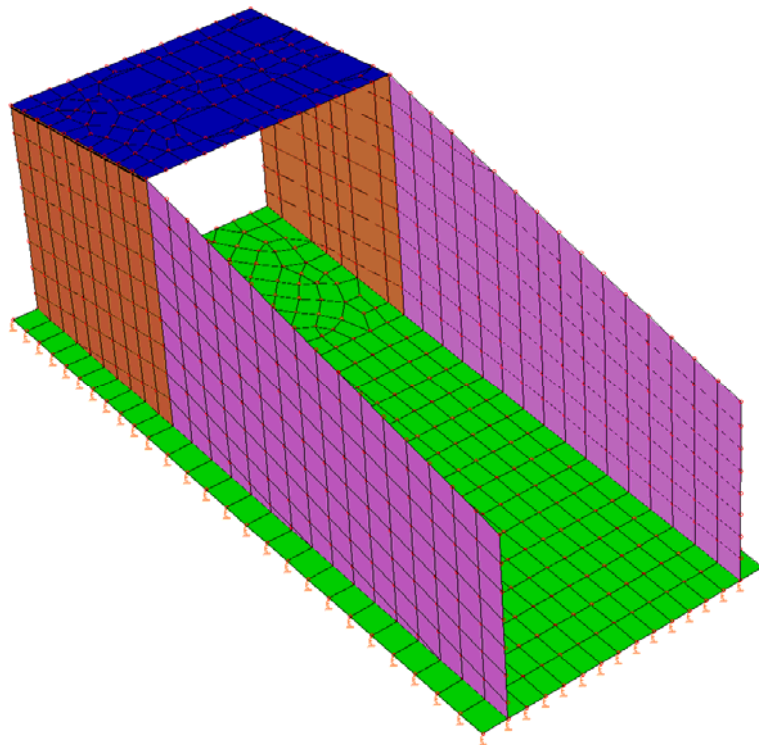
Viste prospettive del tombino agli elementi finiti (solida e unifilare)
