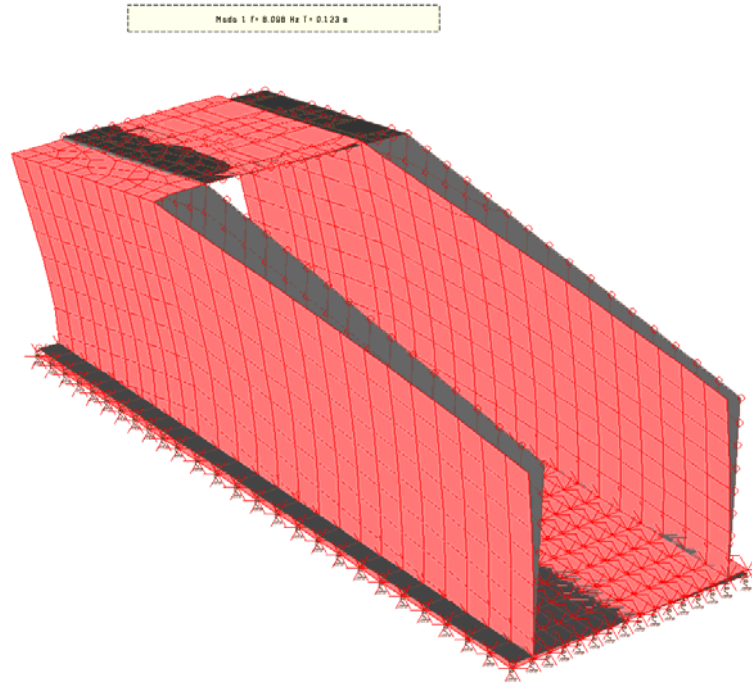
1° Modo di vibrare – principale in x-x
