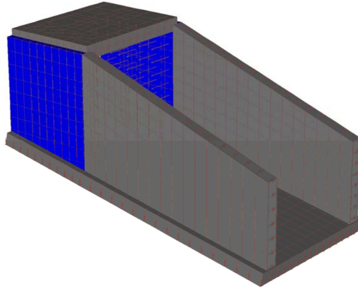
Condizione di carico n°7 (in colore blu le superfici delle spalle caricate)
