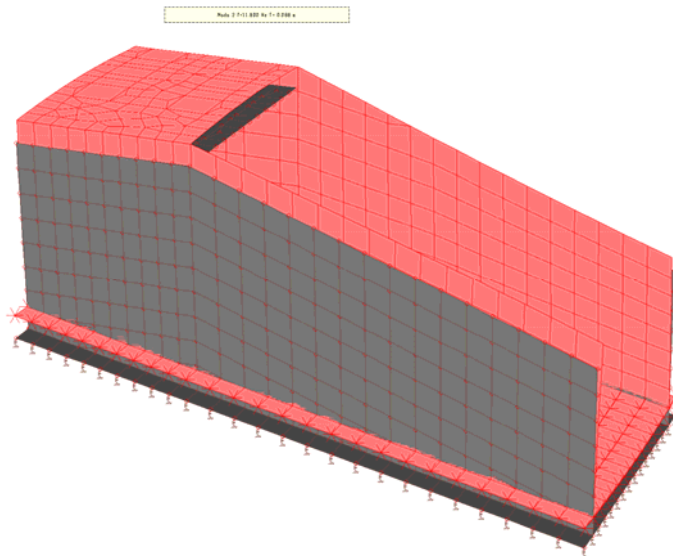
2° Modo di vibrare – principale in z-z
