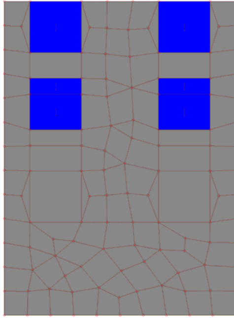
Condizione di carico n°5 (in colore blu le superfici della soletta caricate)
