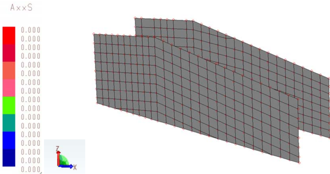
Inviluppo Combinazioni SLU e SLV – armature superiori aggiuntive lungo x [kg/cmq] (ferri orizzontali)
