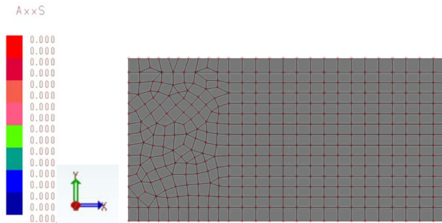
Involuppo Combinazioni SLU e SLV – armature superiori aggiuntive lungo x [kg/cmq]
