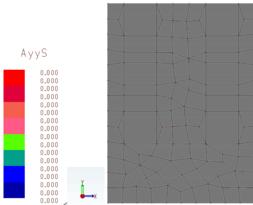
Inviluppo Combinazioni SLU e SLV – armature superiori aggiuntive lungo y [kg/cmq]
