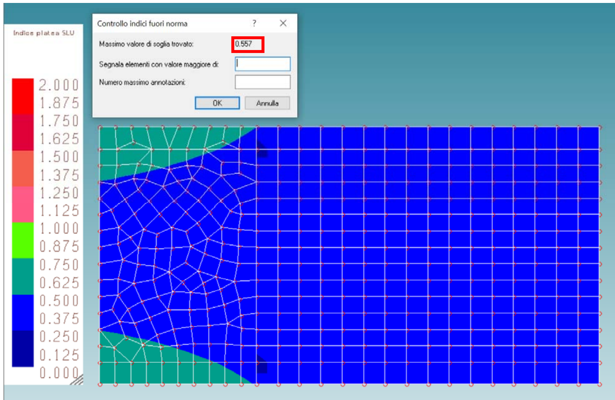
Inviluppo Combinazioni agli SLV – indici di resistenza del qlim della fondazione (sismici)
