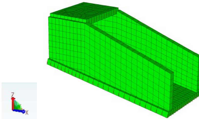
Verifica degli elementi guscio costituenti il modello FEM
