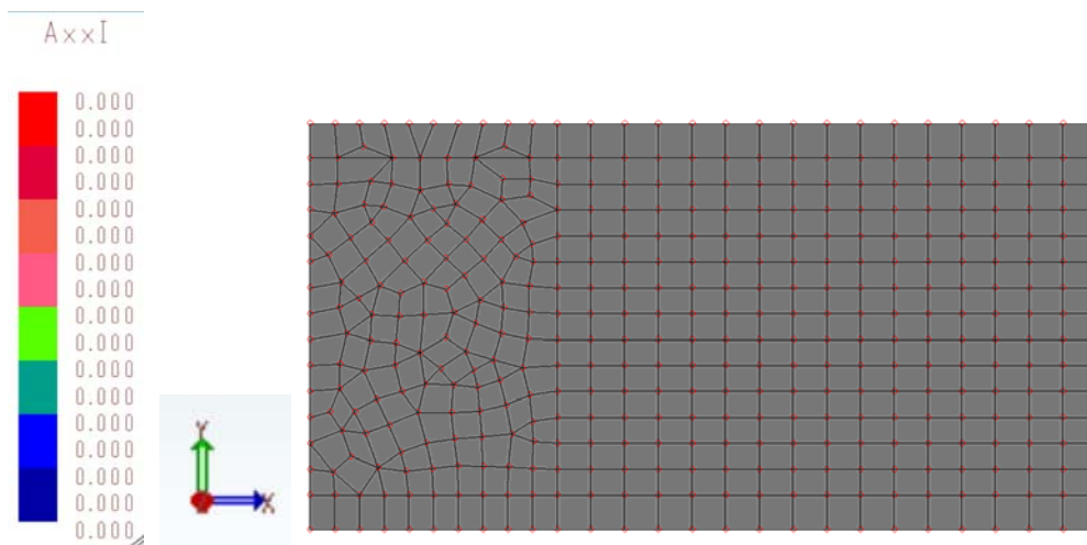
Involuppo Combinazioni SLU e SLV – armature inferiori aggiuntive lungo x [kg/cmq]
