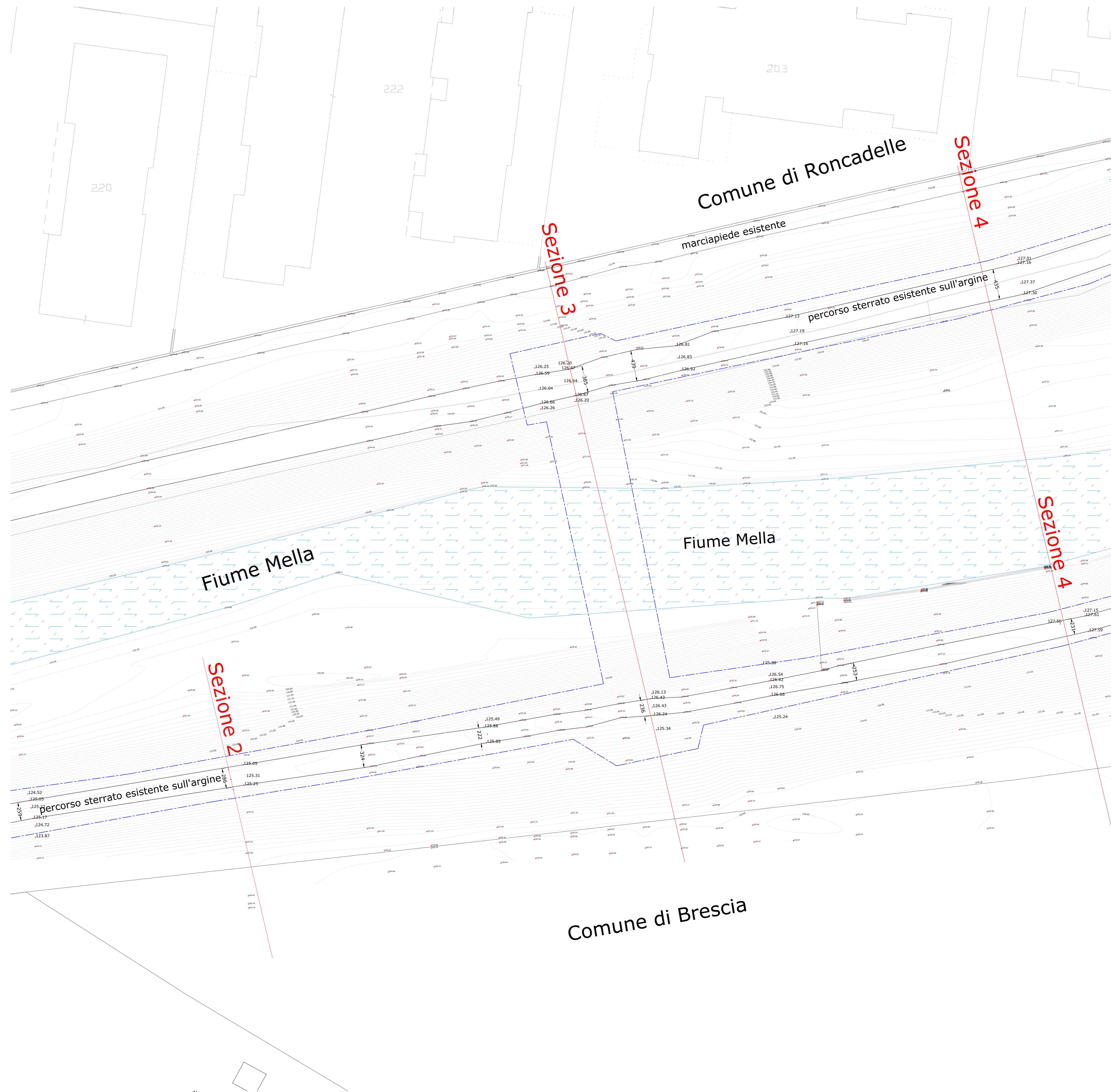
PIANTA - quadro B - scala 1:200
