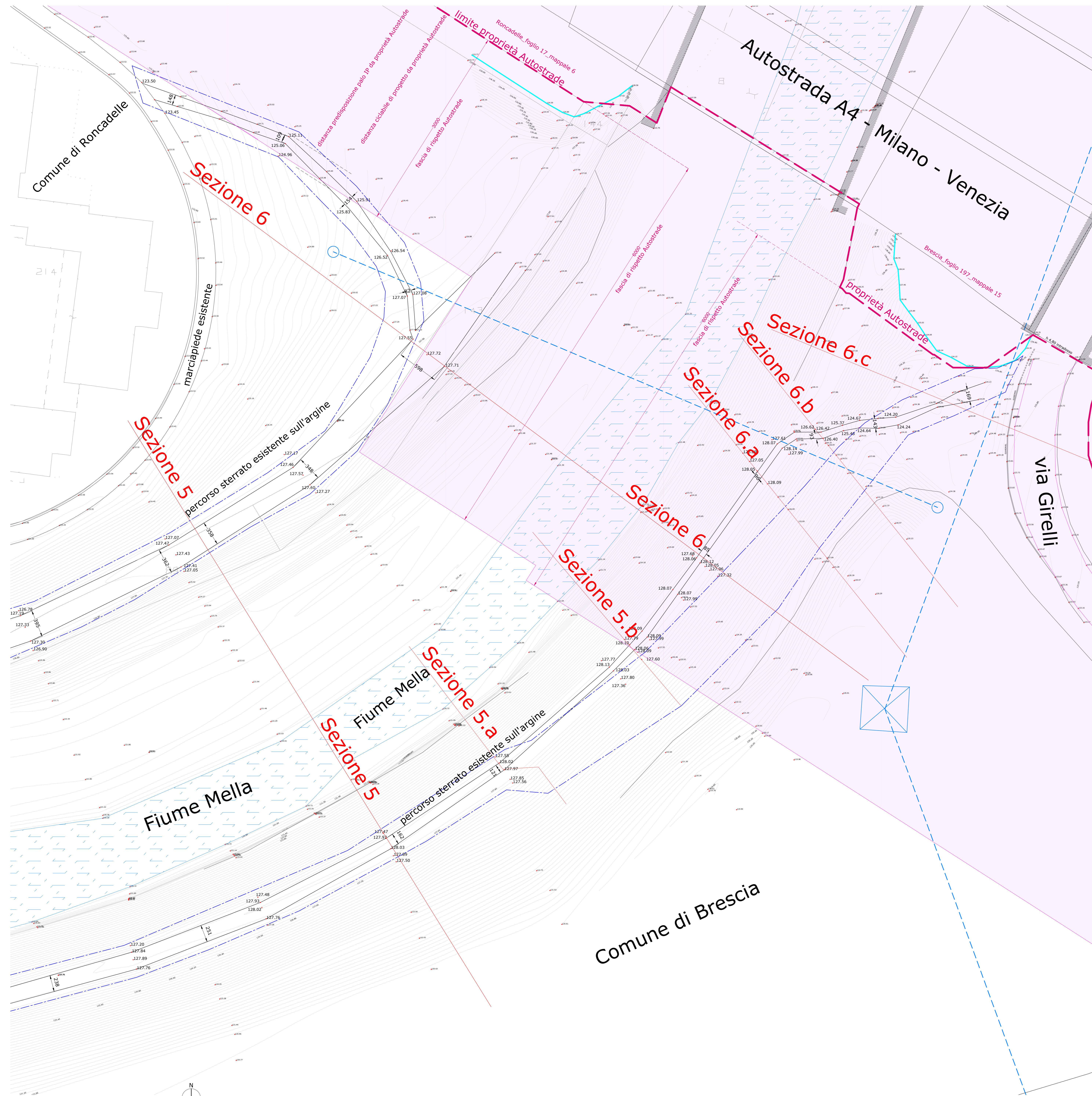
PIANTA - quadro A - scala 1:200
