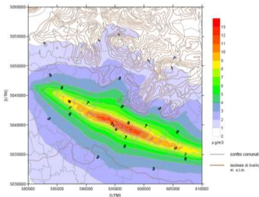
Figura 14 - Concentrazione media annuale di PM10 ( \mu\text{g}/\text{m}^3 ) attribuibile al solo traffico veicolare (parco circolante al 2000).
