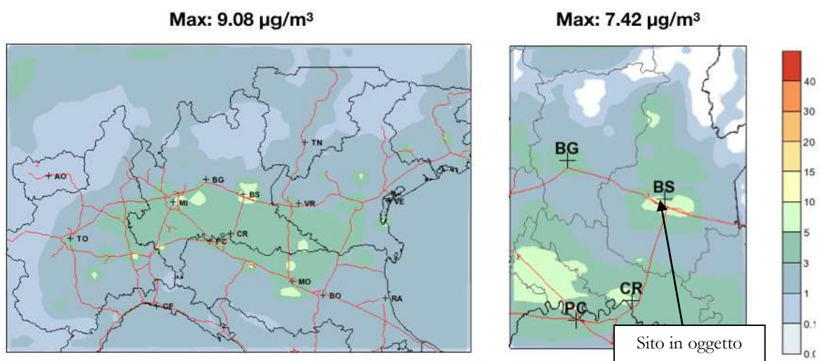
Figura 4.21: Impatto del gruppo S-A "Agricoltura" sulla concentrazione media annuale di PM10 ( \mu\text{g}/\text{m}^3 ).
