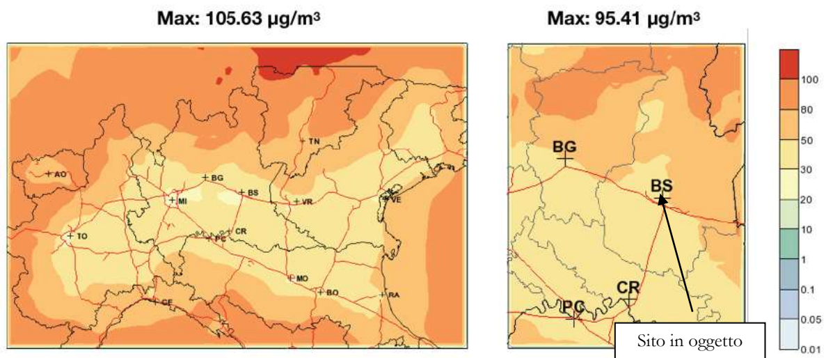
Figura 4.1: Impatto del gruppo S-A "Condizioni al contorno" sulla concentrazione media annuale di O 3 (µg/m 3 )
