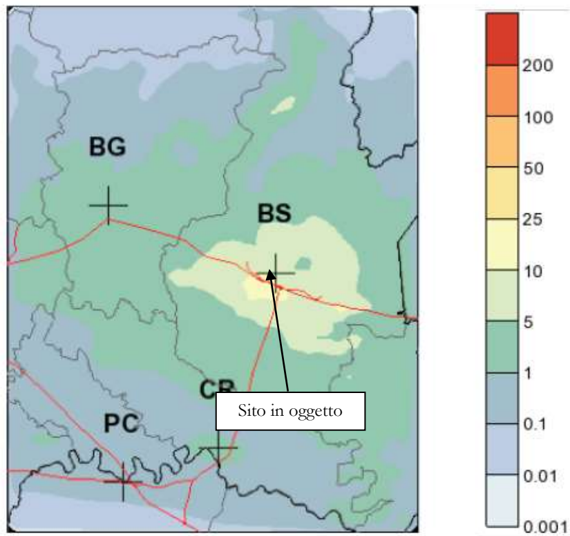
Figura 5.11: Concentrazione media annuale di PCB-TOT (pg/m 3 ).
