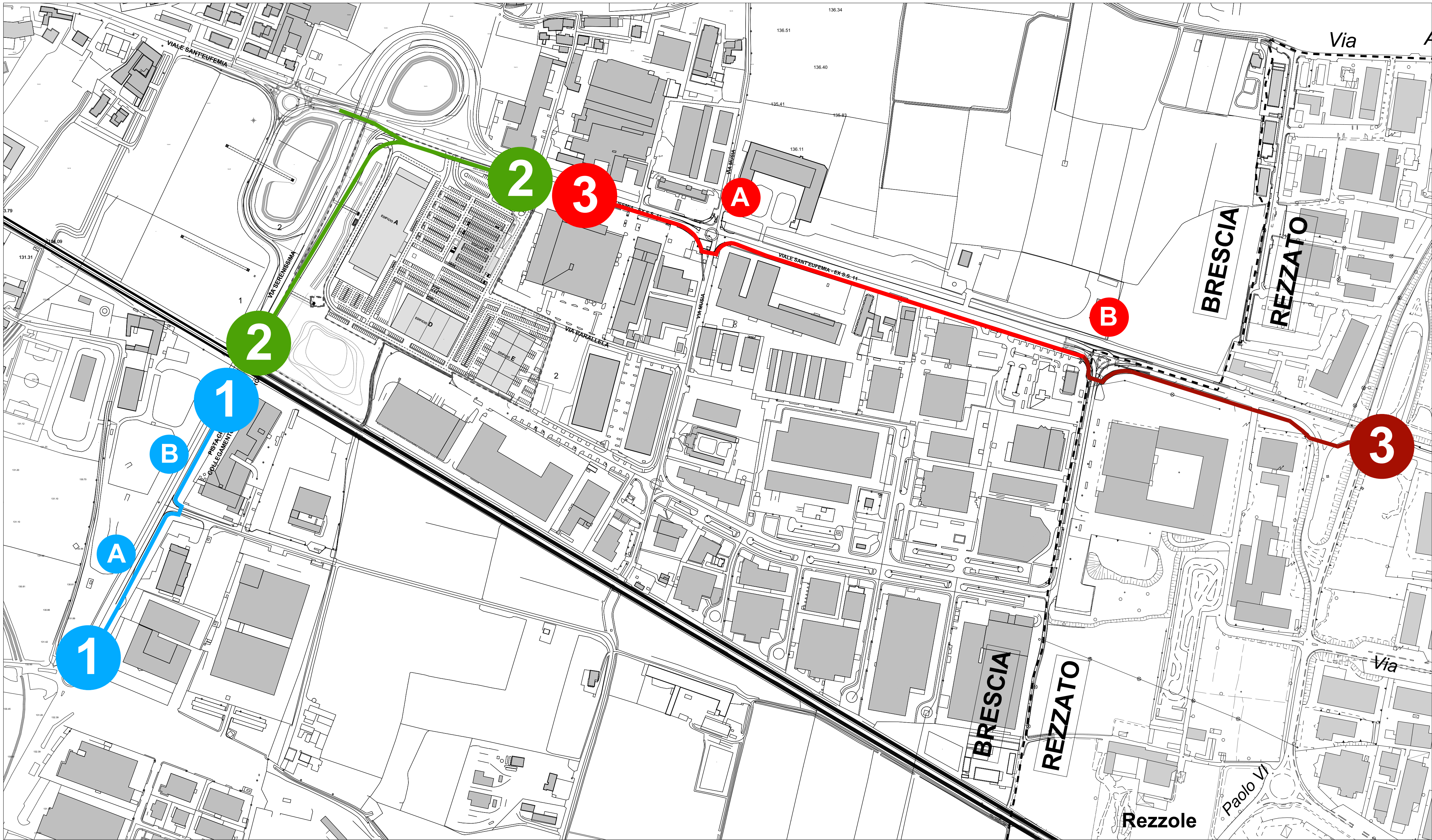
PISTA CICLABILE - VISIONE D'INSIEME
