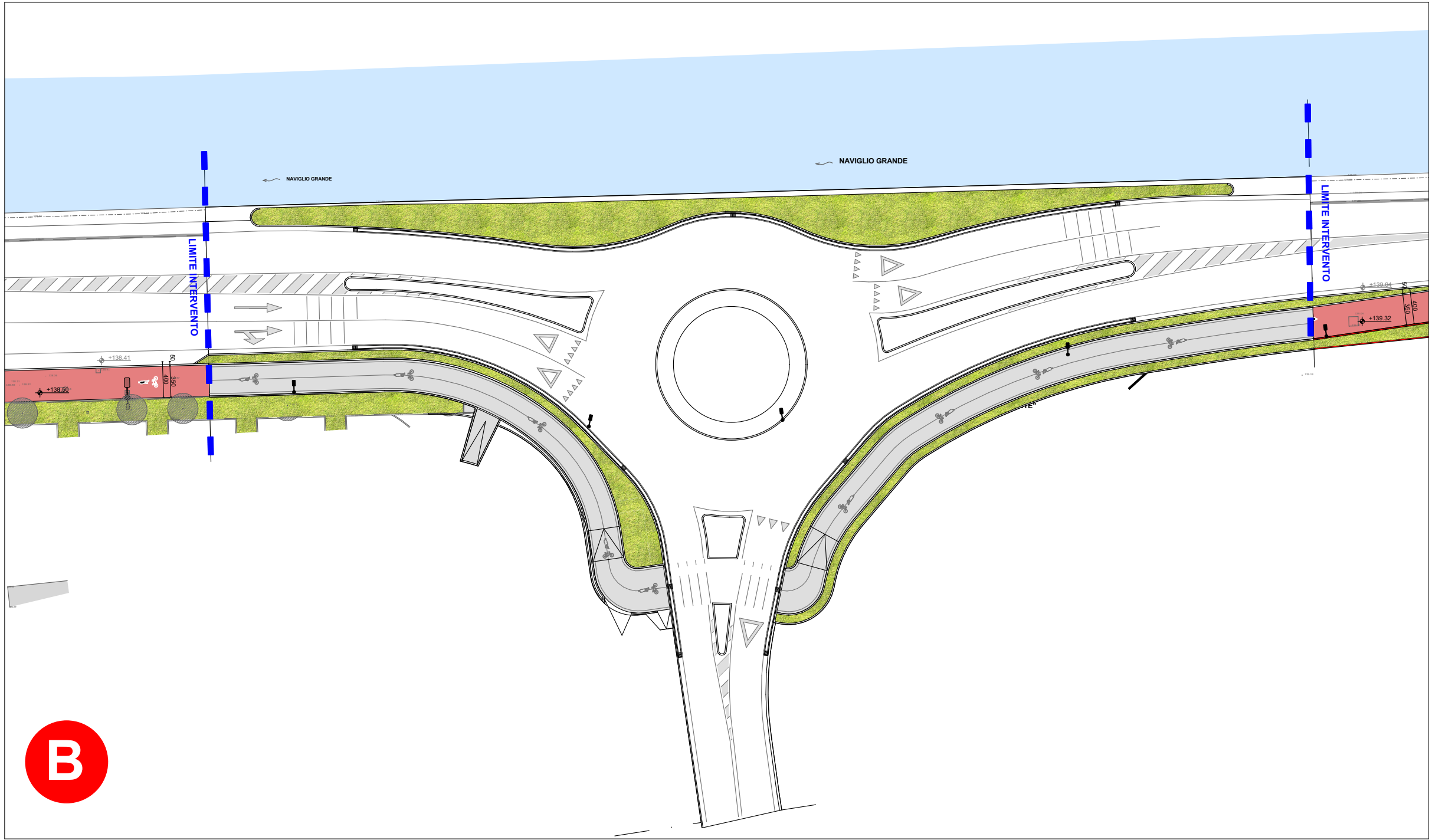
ROTATORIA VIALE S. EUFEMIA/VIA CHIAPPA (GIÀ REALIZZATA)
