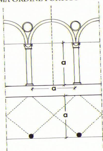
SCHEMA ORDINE PORTICO
