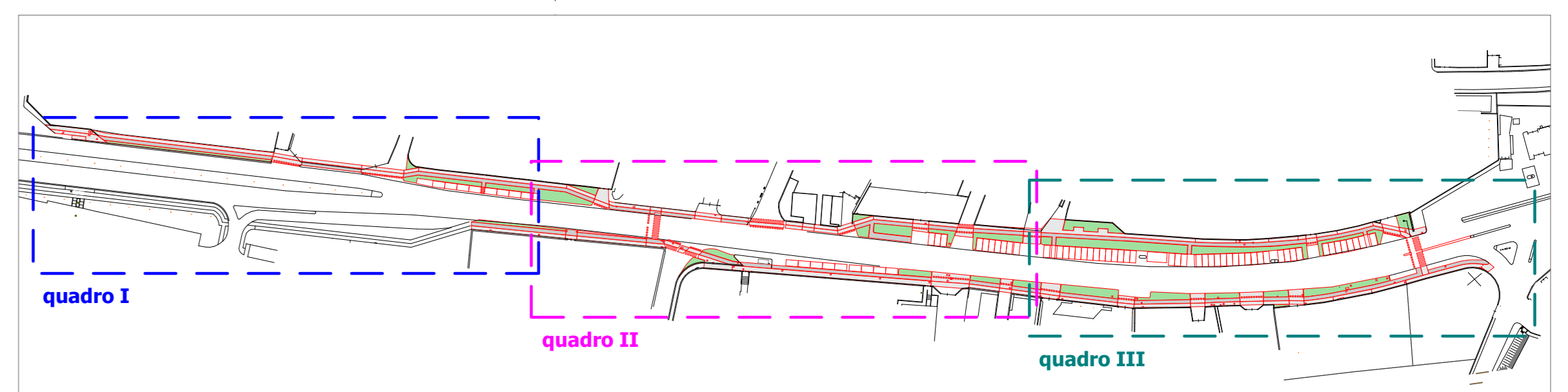
PLANIMETRIA DI RAFFRONTO - QUADRO I scala 1:200
