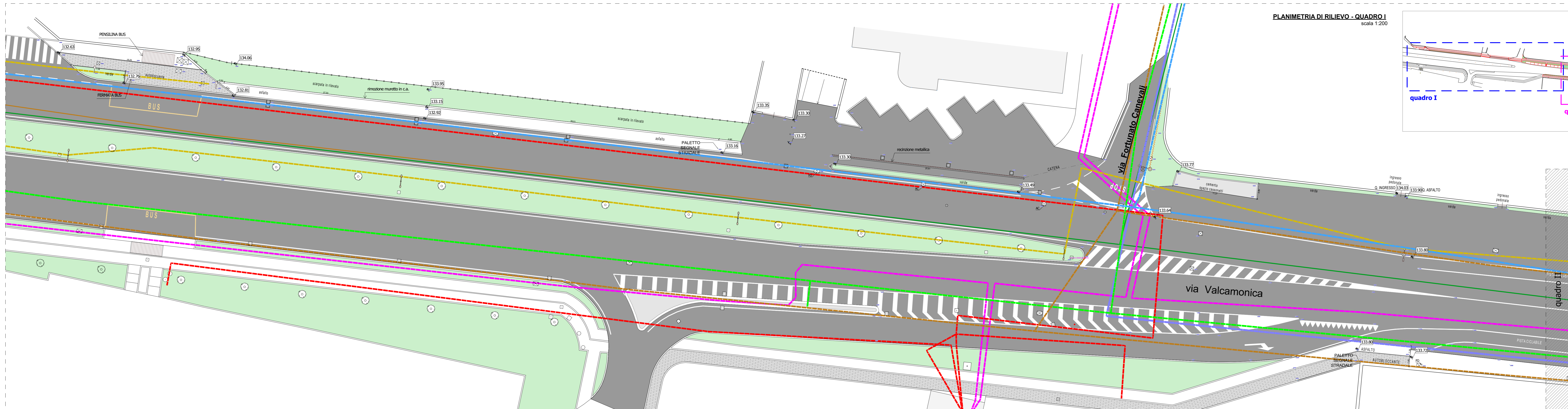
PLANIMETRIA DI RILIEVO - QUADRO II scala 1:200
