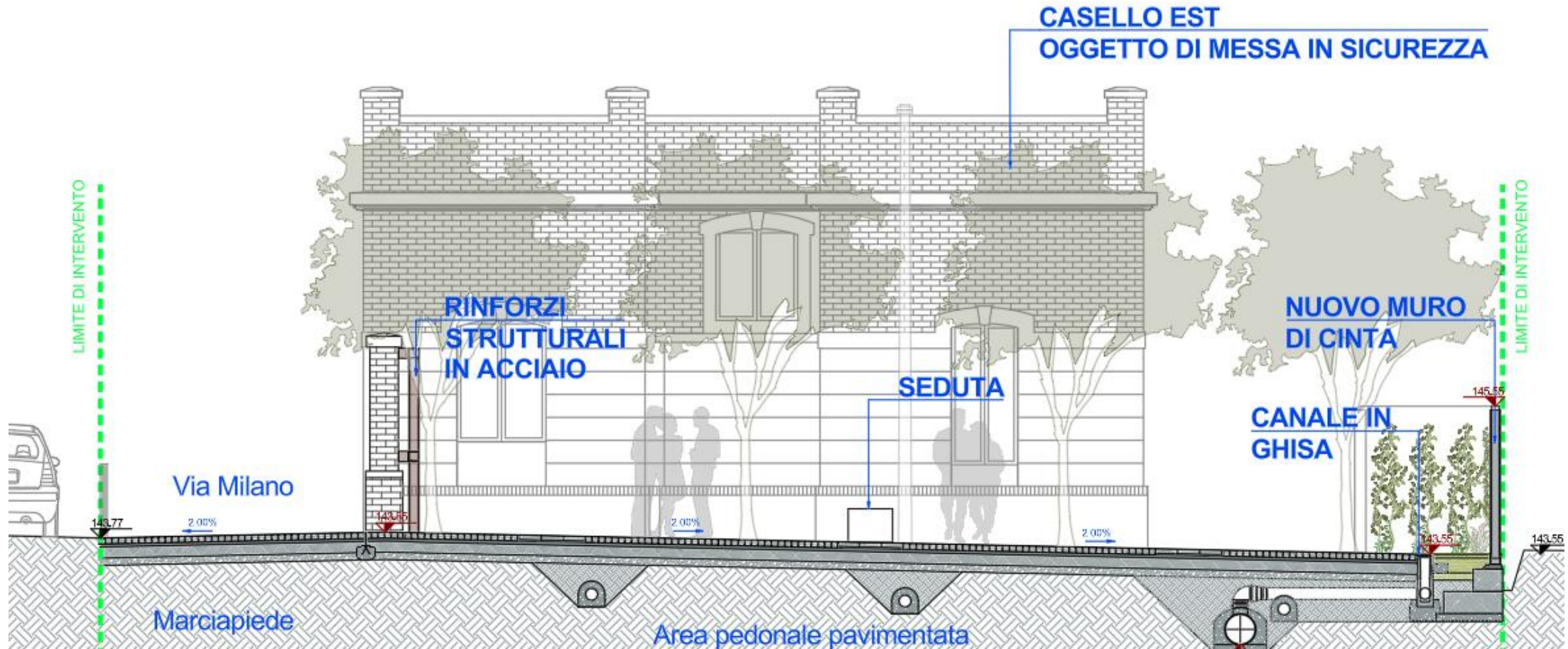
SEZIONE TRASVERSALE SULLA PIAZZA
