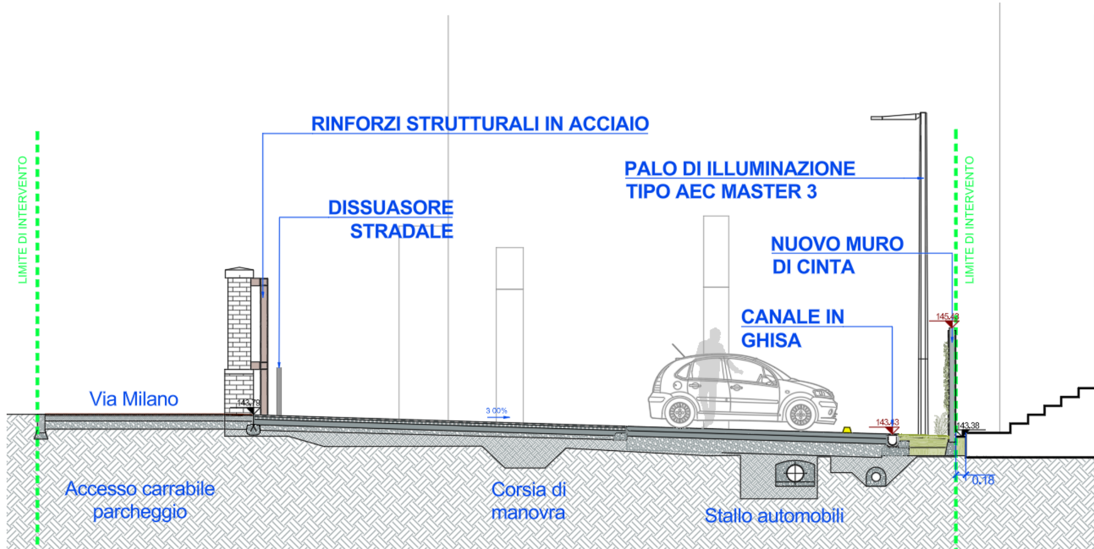
SEZIONE TRASVERSALE SUL PARCHEGGIO EST
