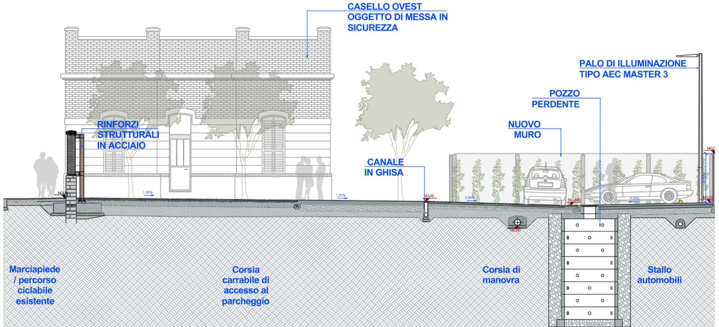
SEZIONE TRASVERSALE SUL PARCHEGGIO OVEST
