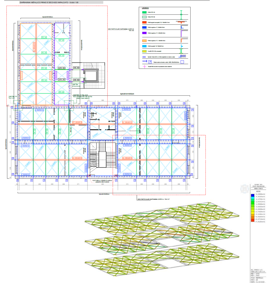
DIAFRAMMA DI PIANO
