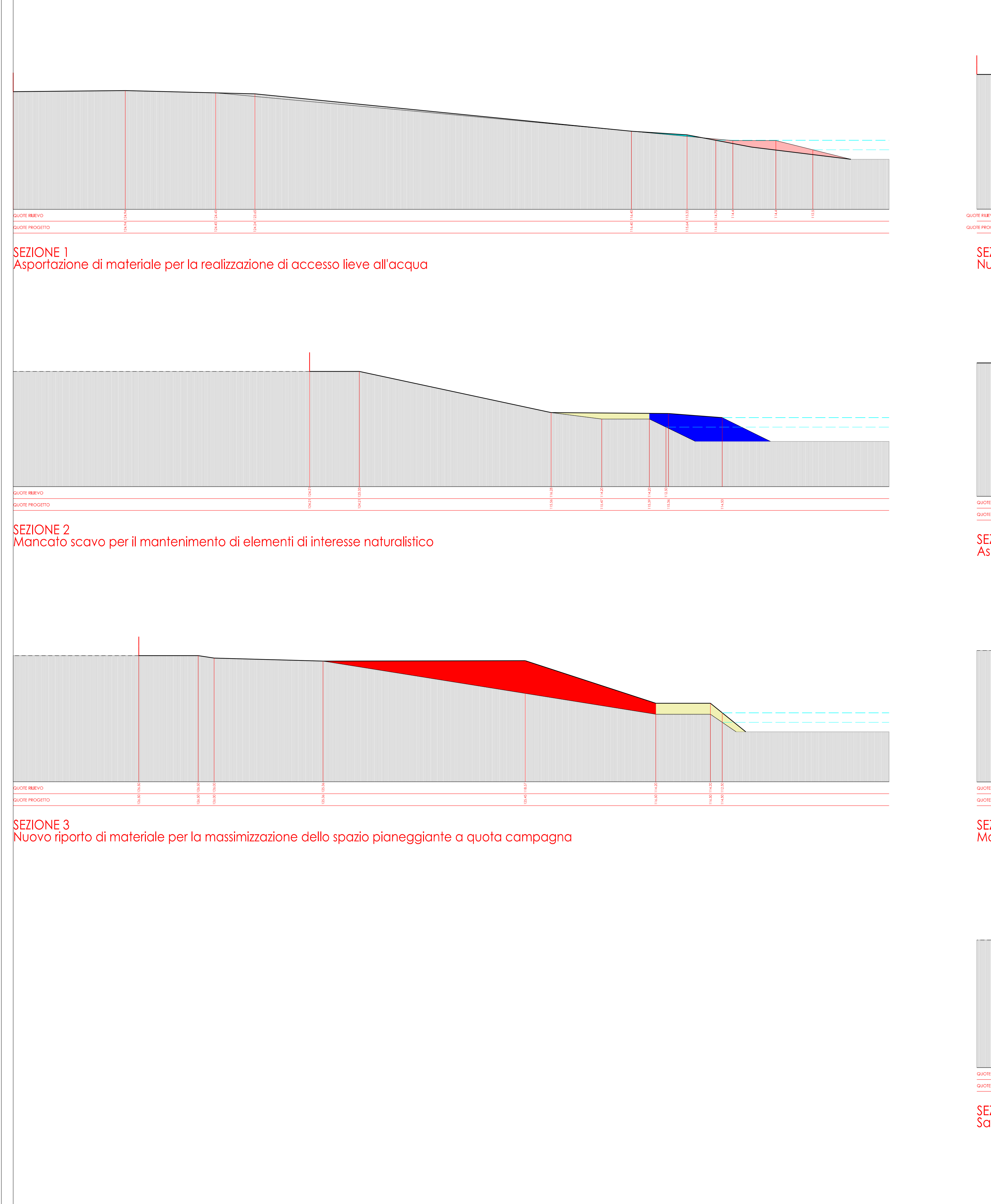
SEZIONI DI DETTAGLIO - scala 1:500
