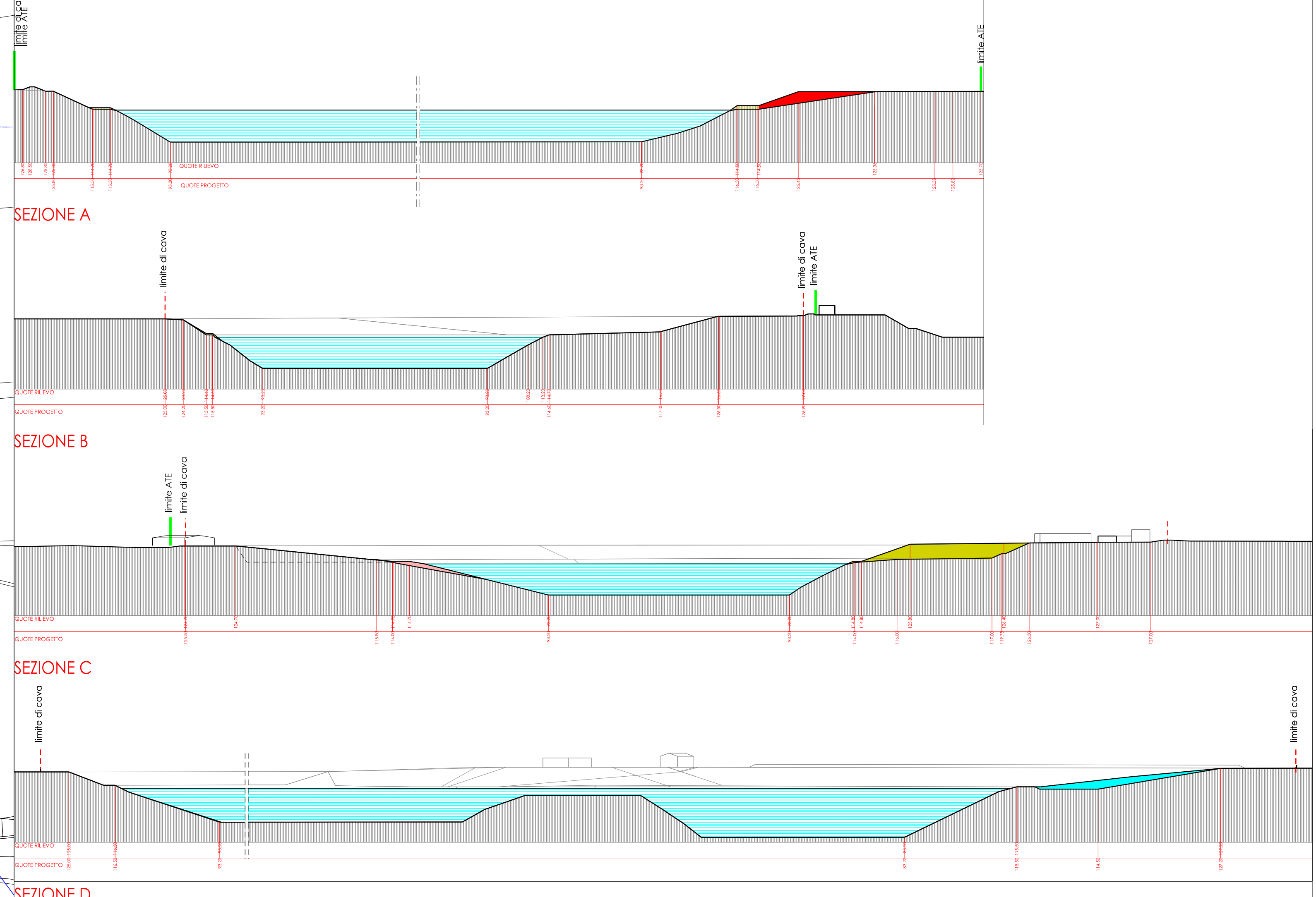
SEZIONI AMBIENTALI - scala 1:2.000
