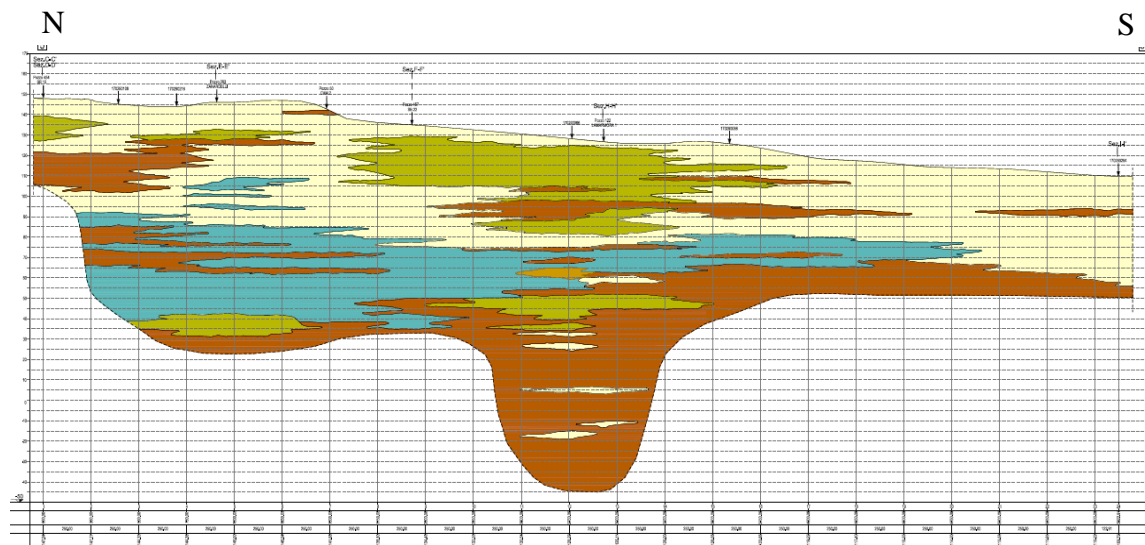
Figura 54: Schema stratigrafico della pianura bresciana
